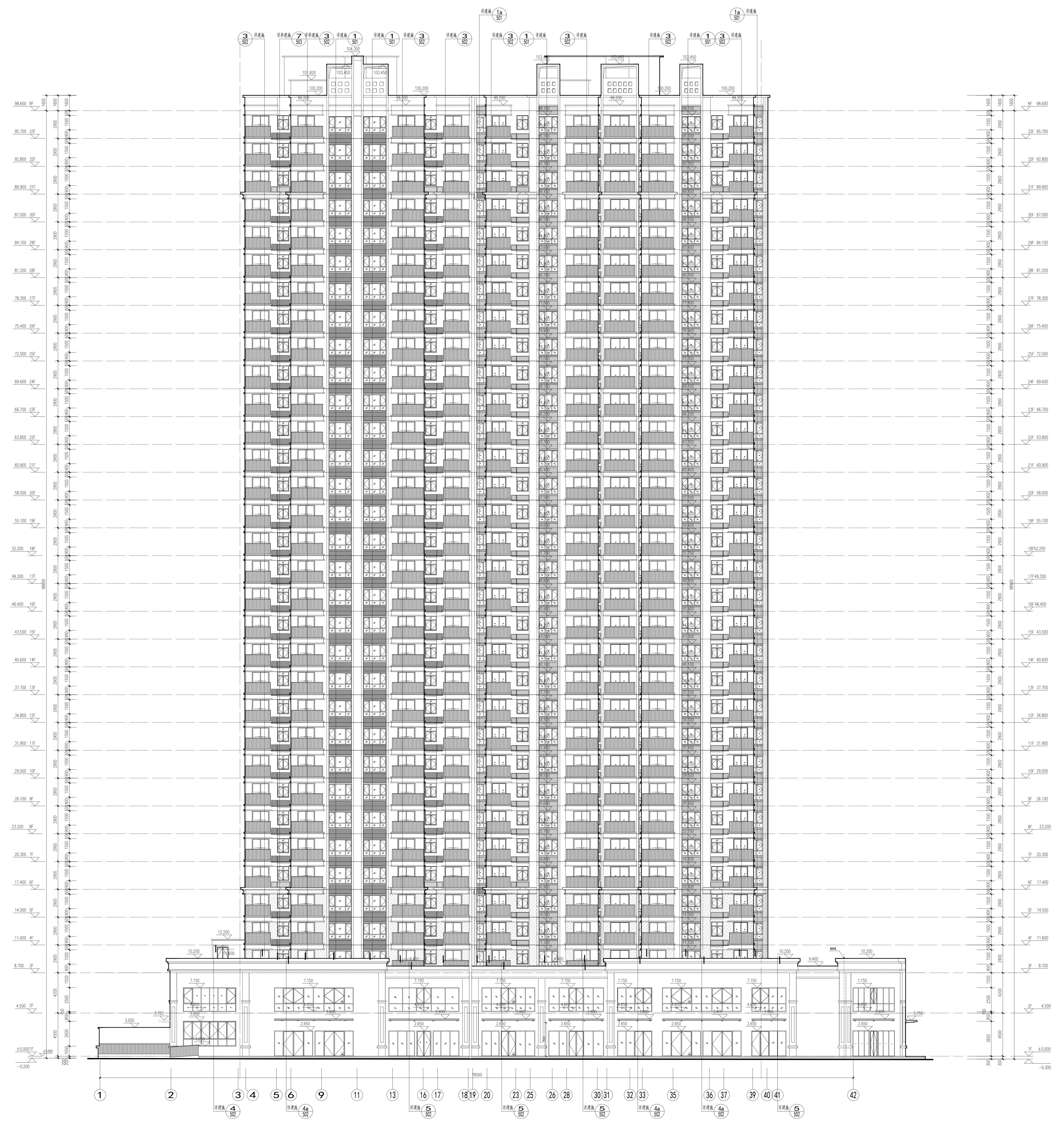
1-42轴立面图 1:150
