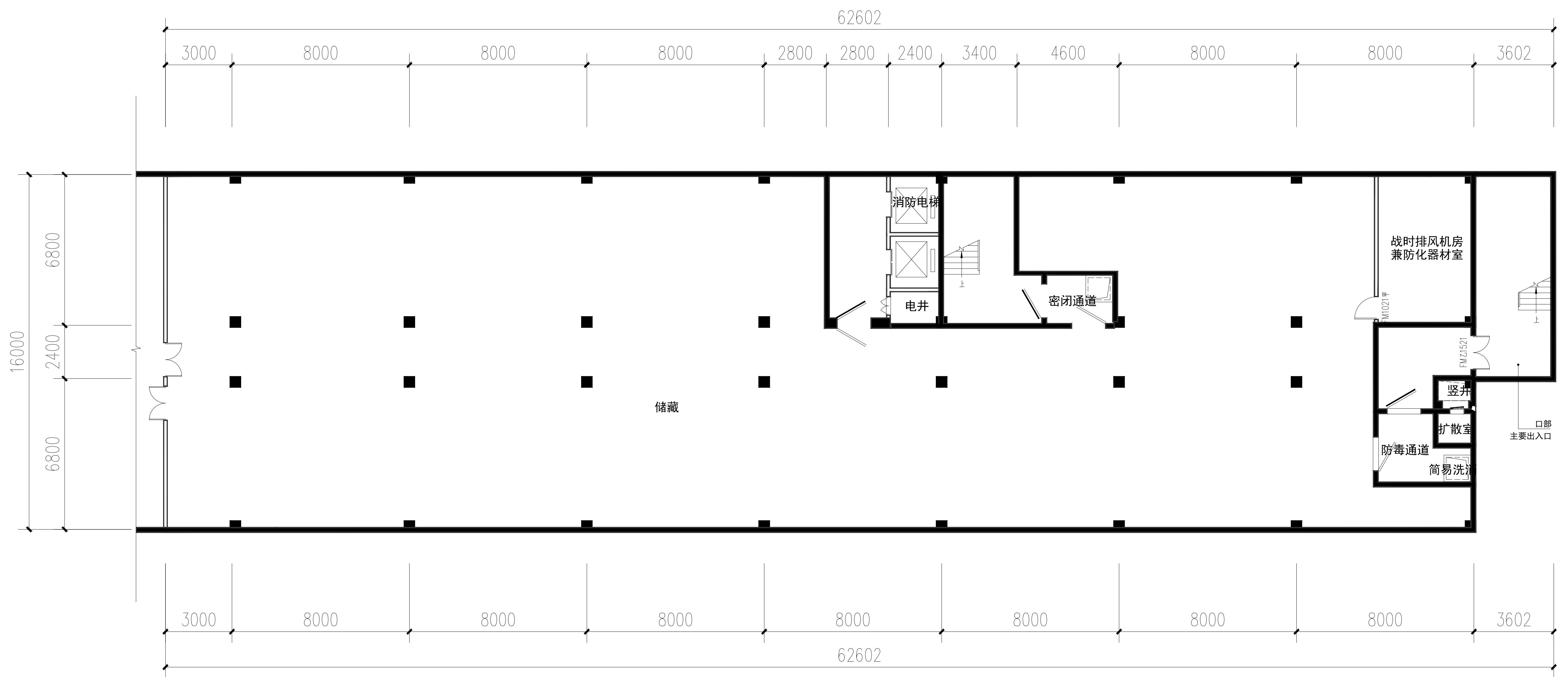
地下一层平面图 1:100
