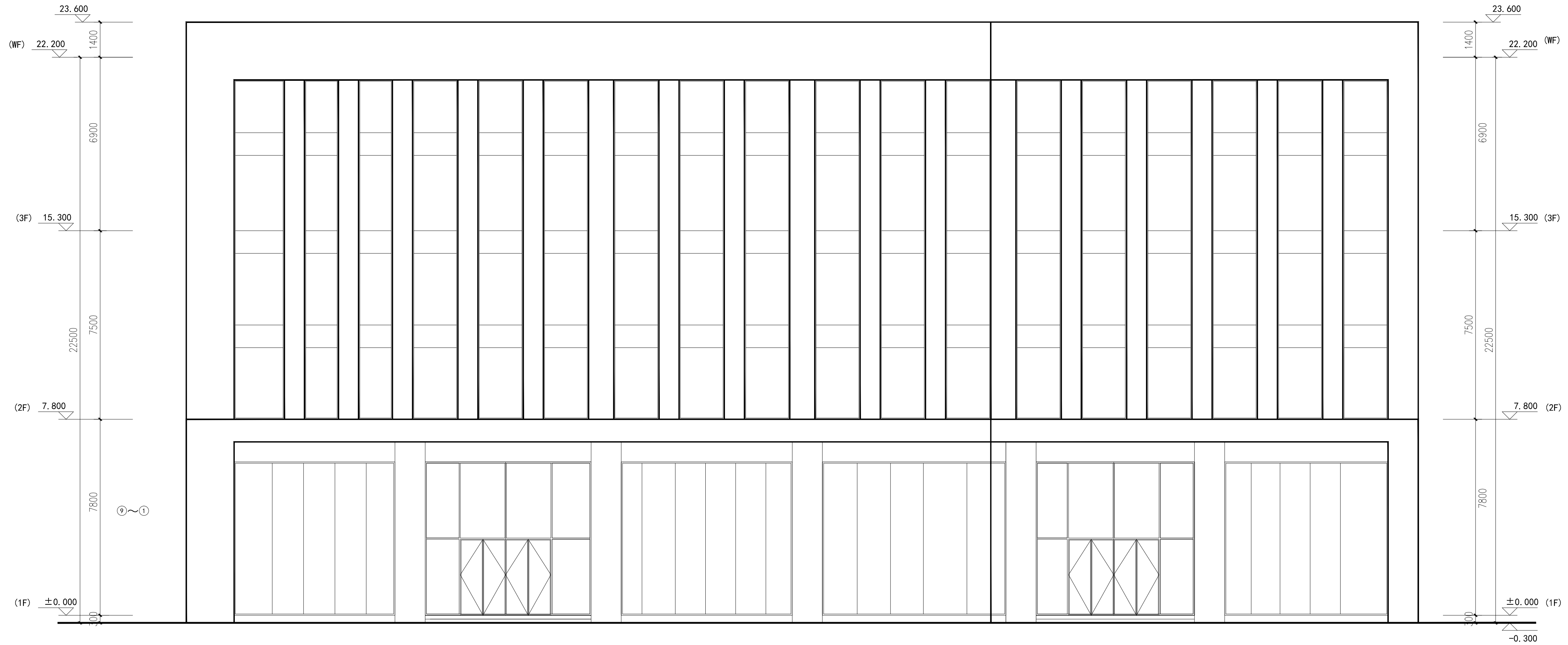
北立面图 1:100
