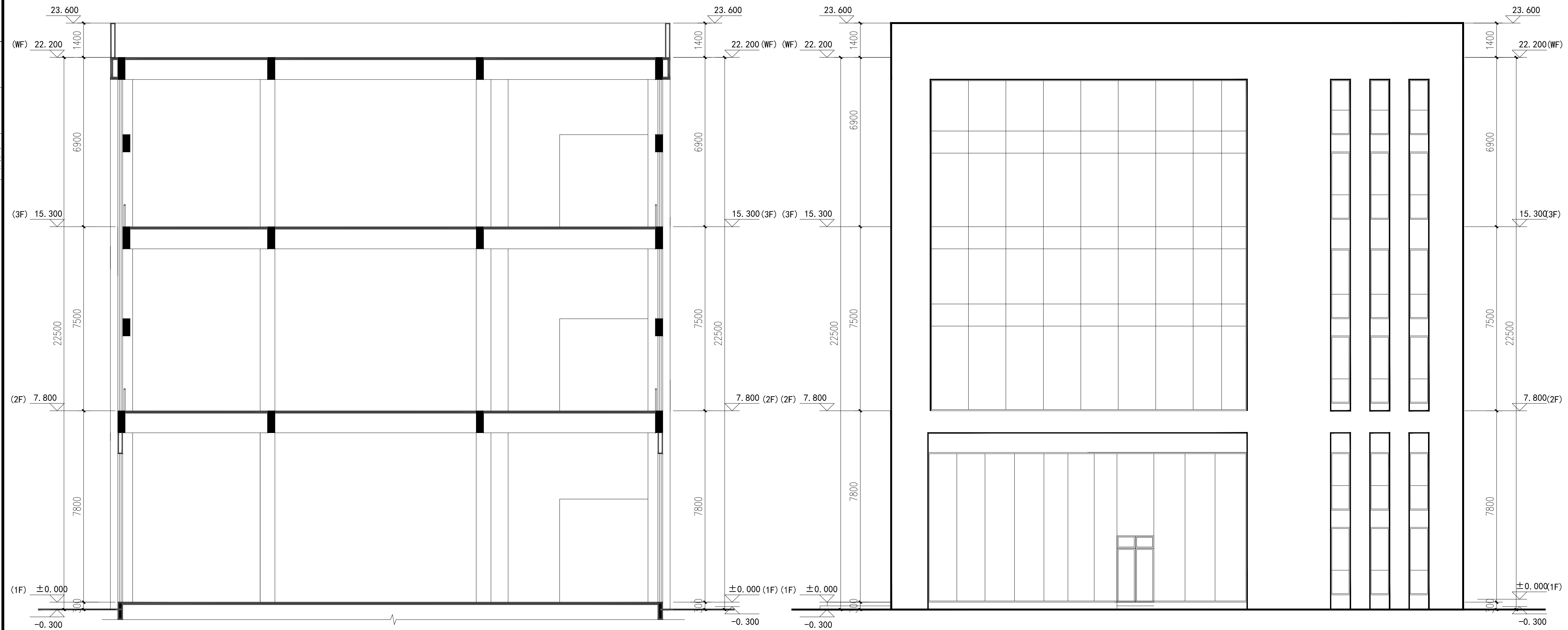
1-1剖面图 1:100
