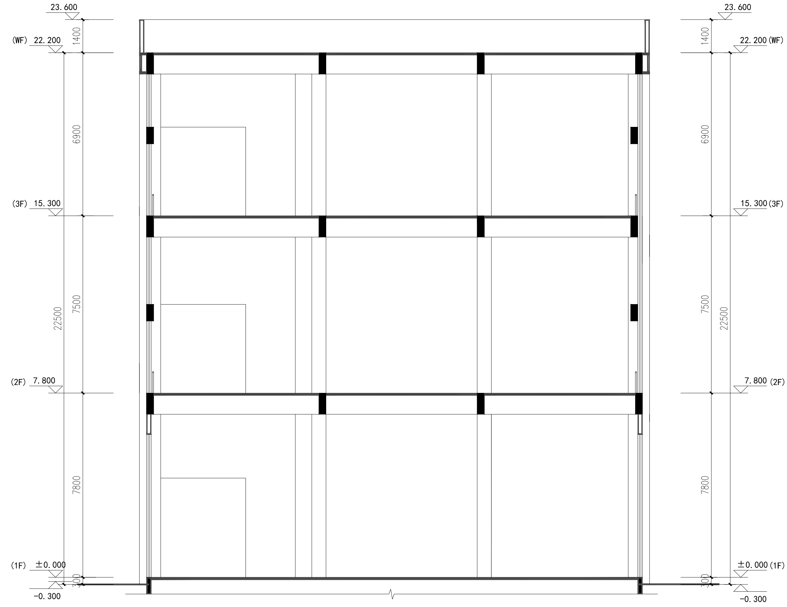
1-1剖面图 1:100
