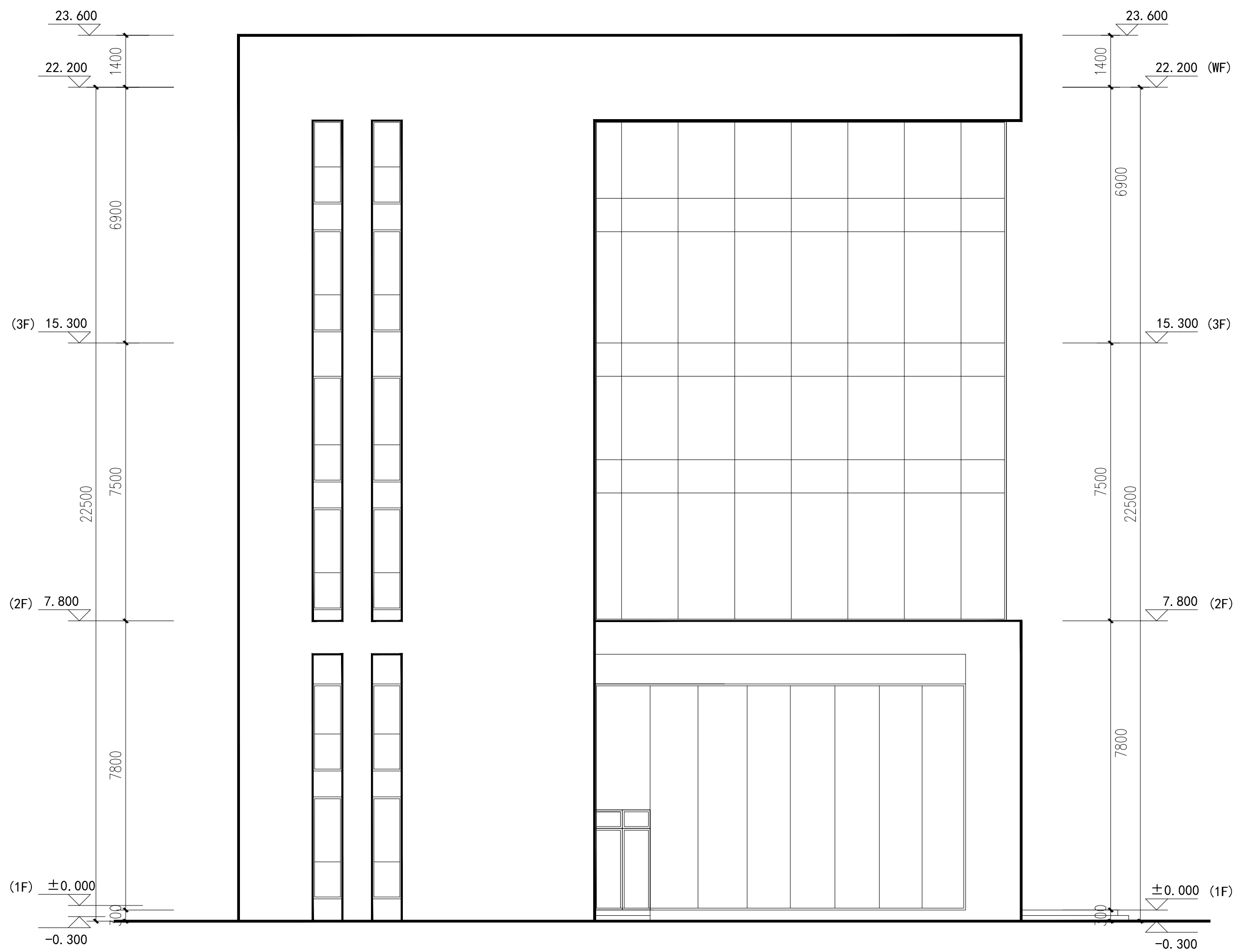
西立面图 1:100
