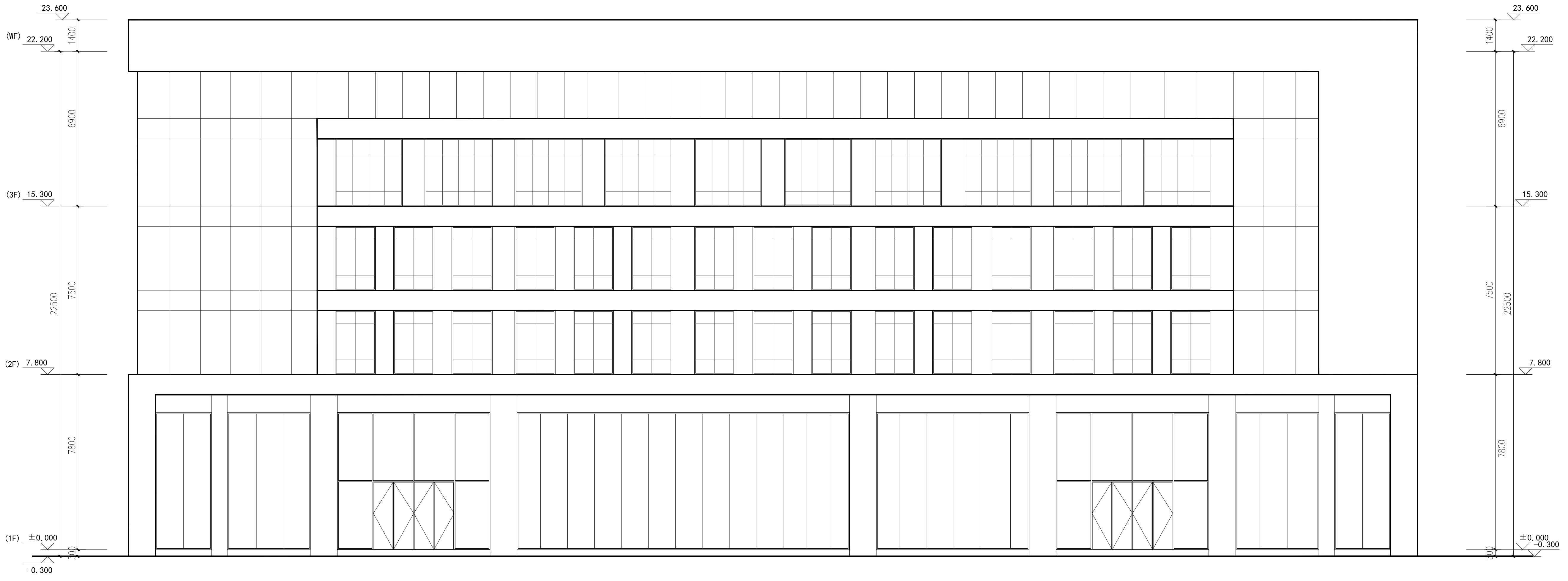
南立面图 1:100
