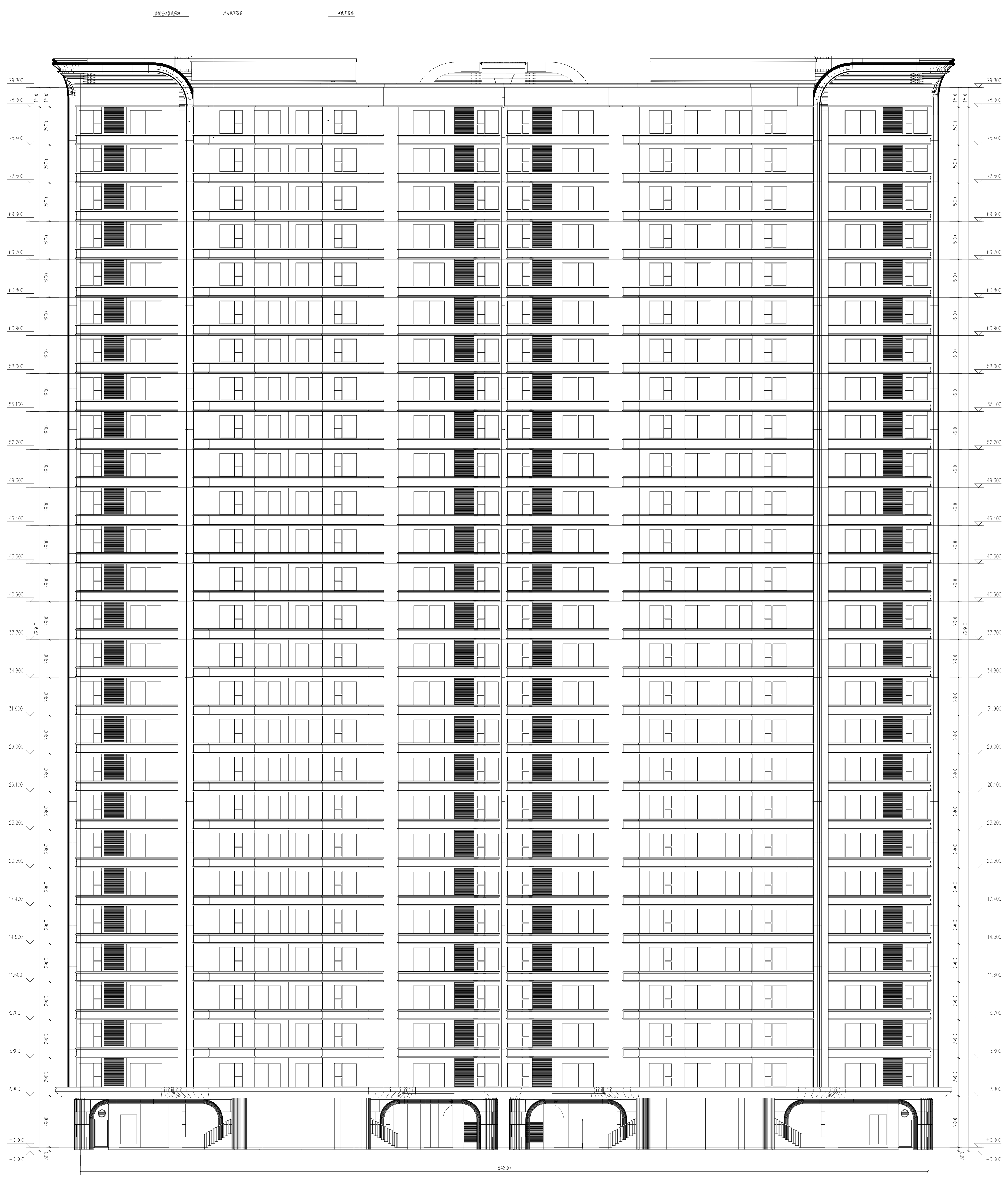
南立面图 1:100
