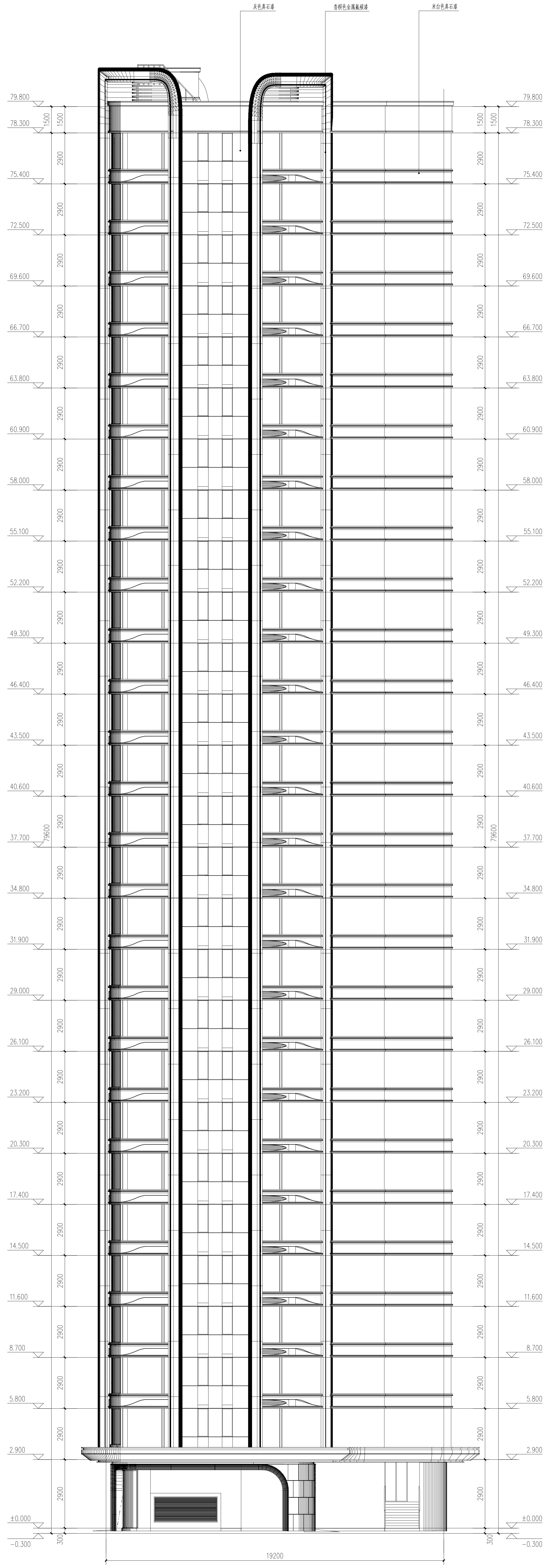
西立面图 1:100
