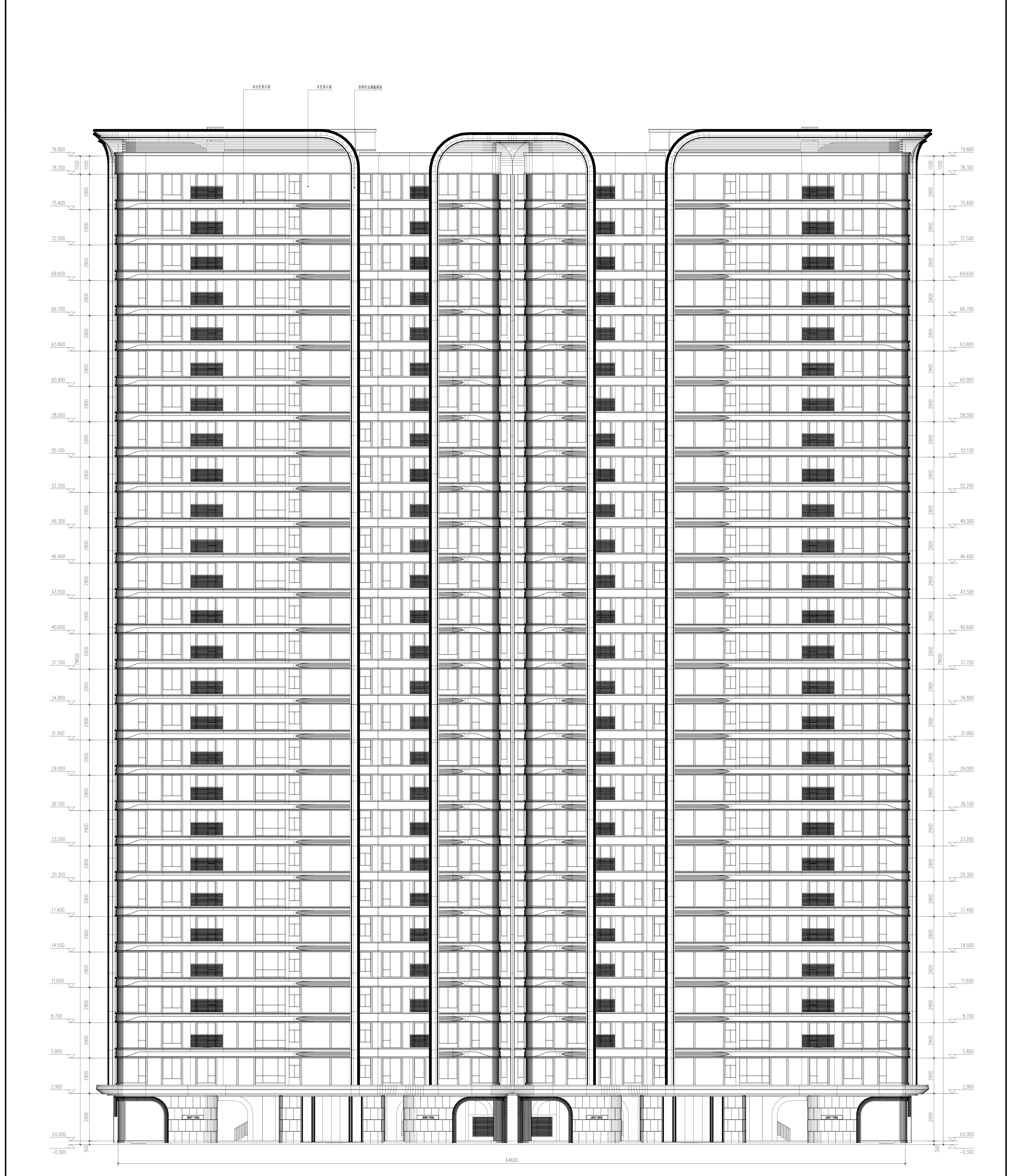
北立面图 1:100
