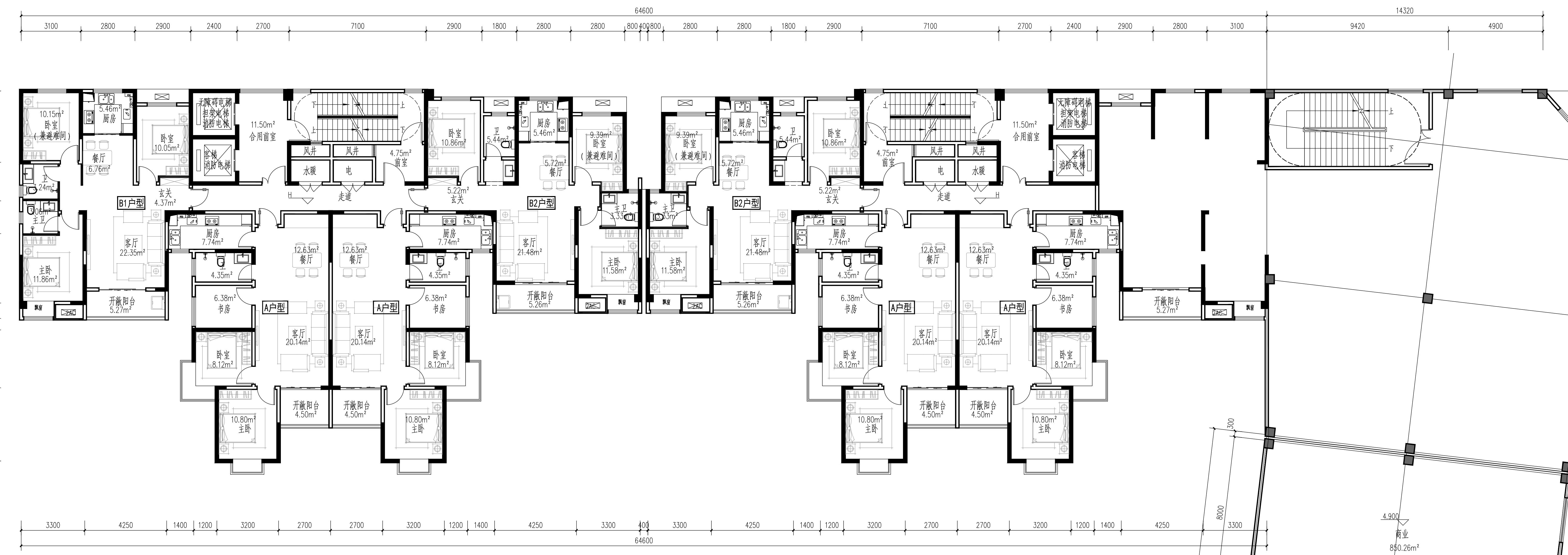
二层平面图 1:100
