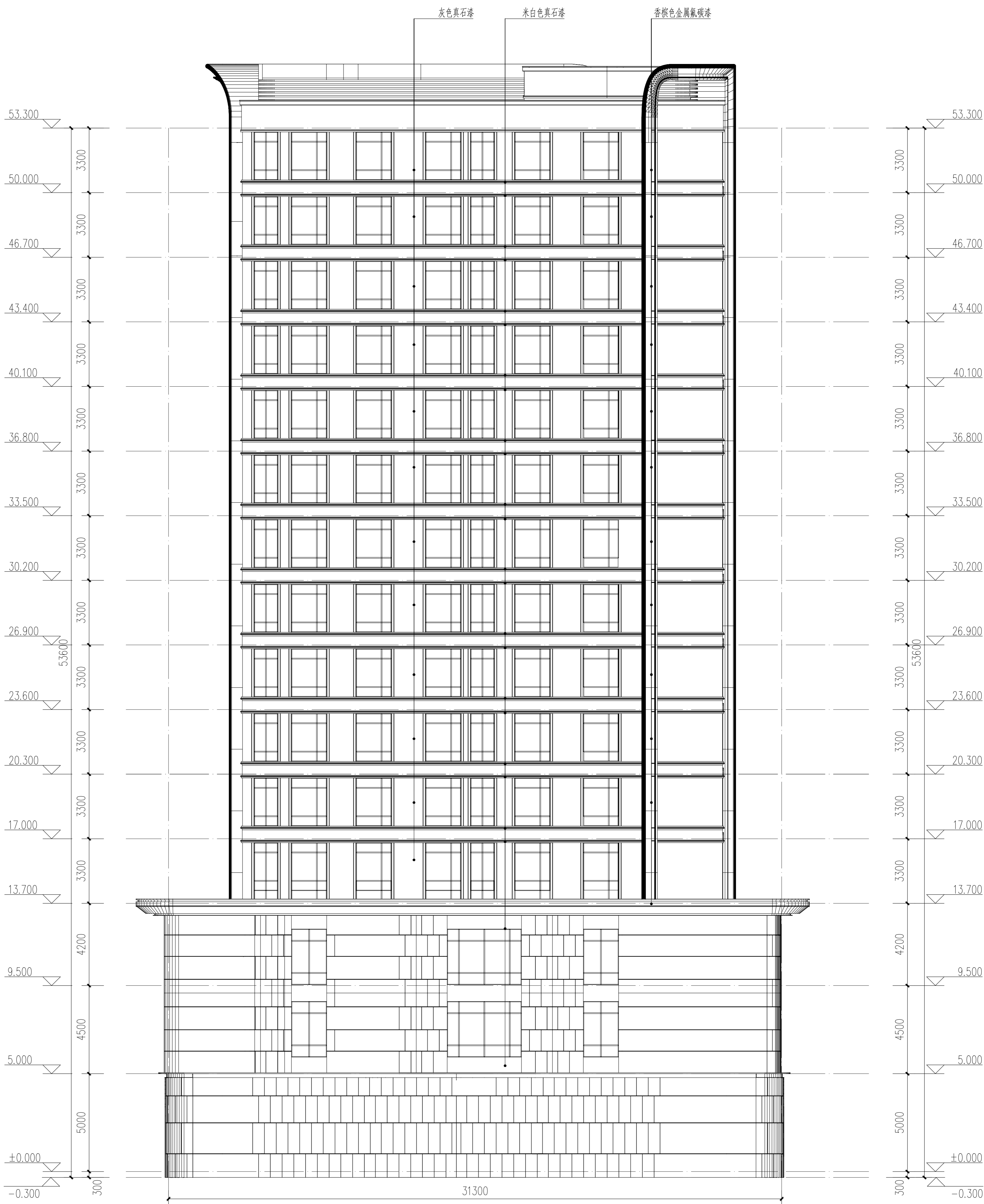
东立面图
