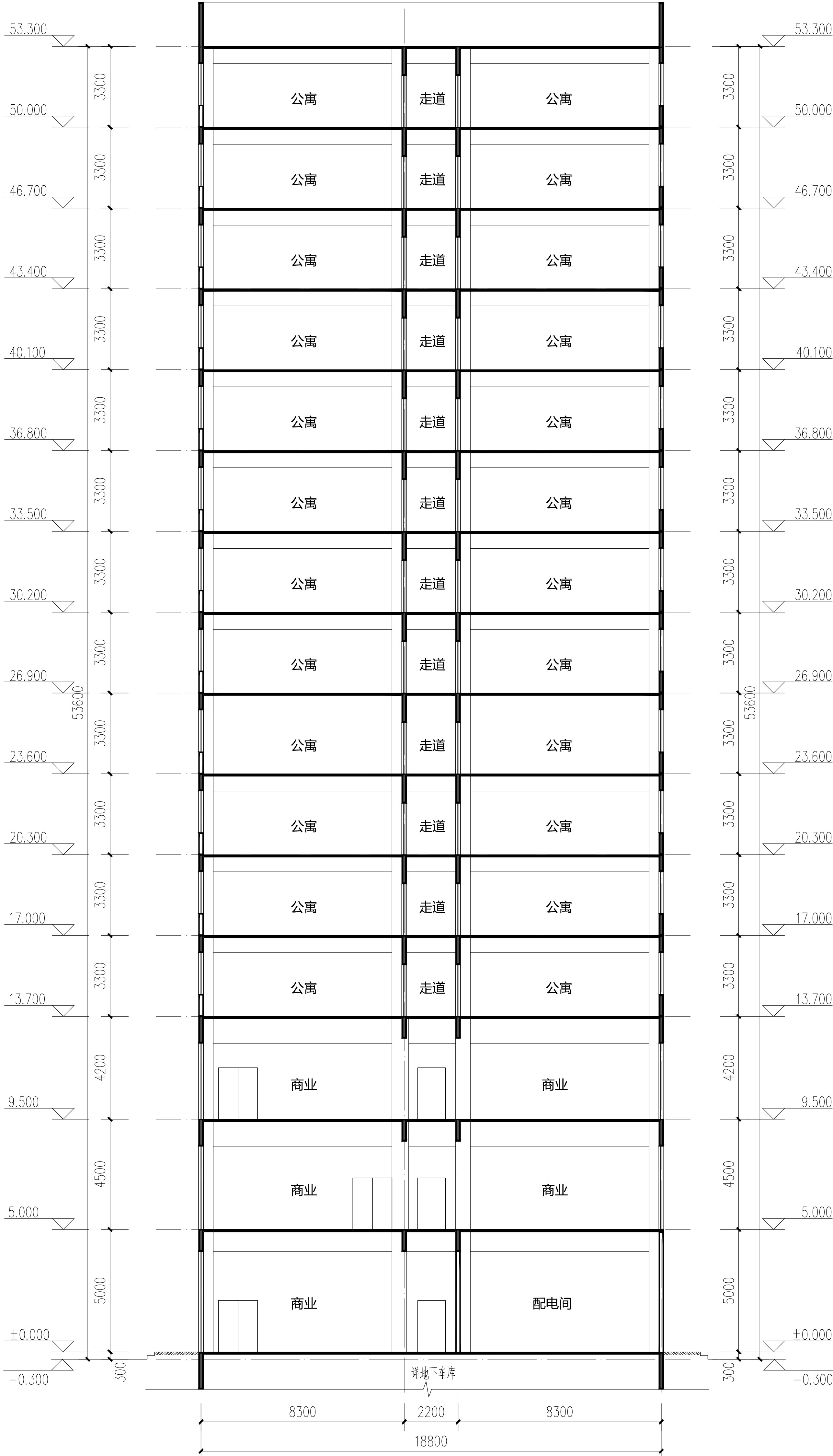
1-1剖面图
