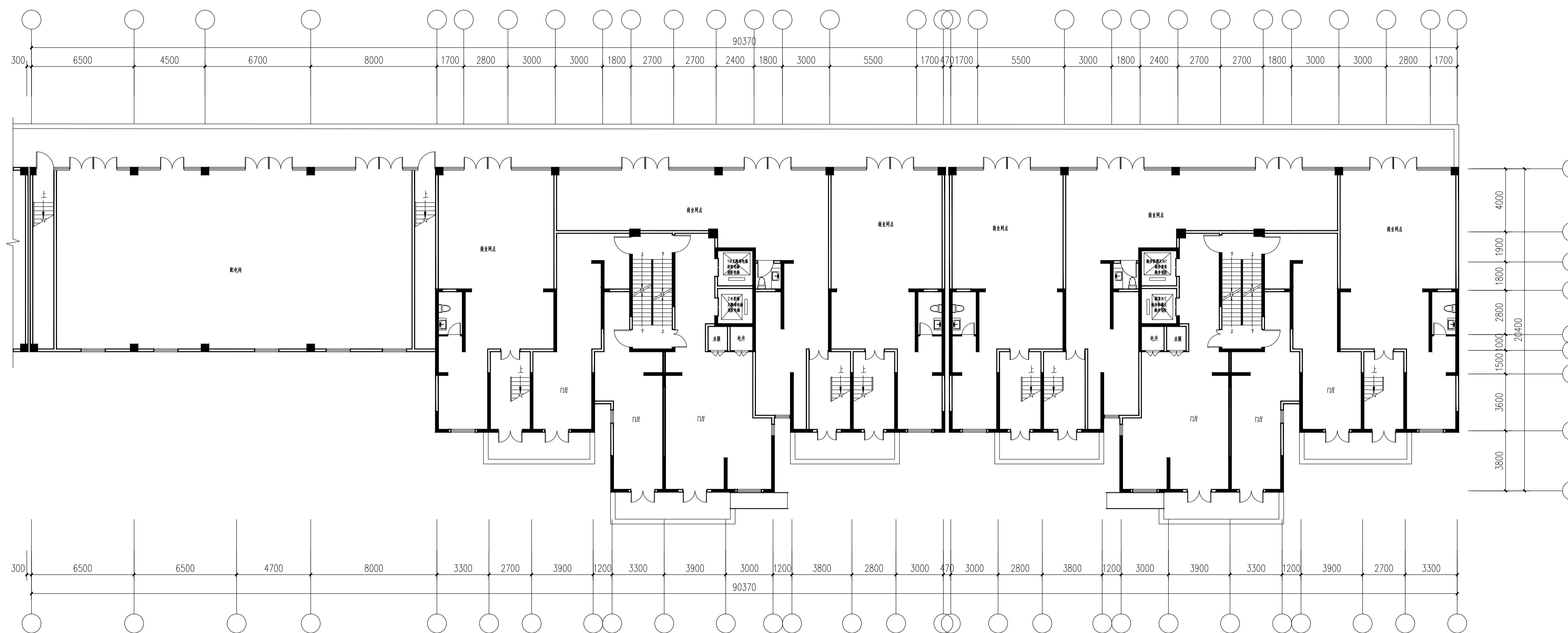
一层平面图
