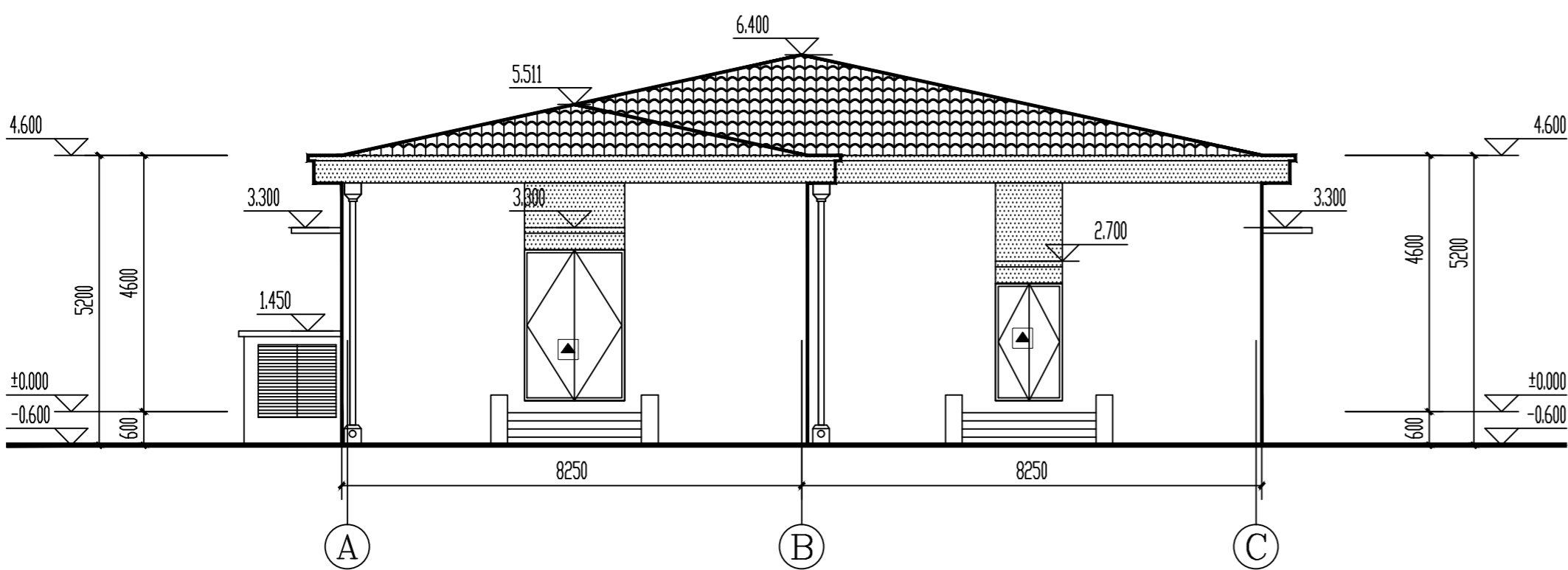
①-③立面图 1:100
