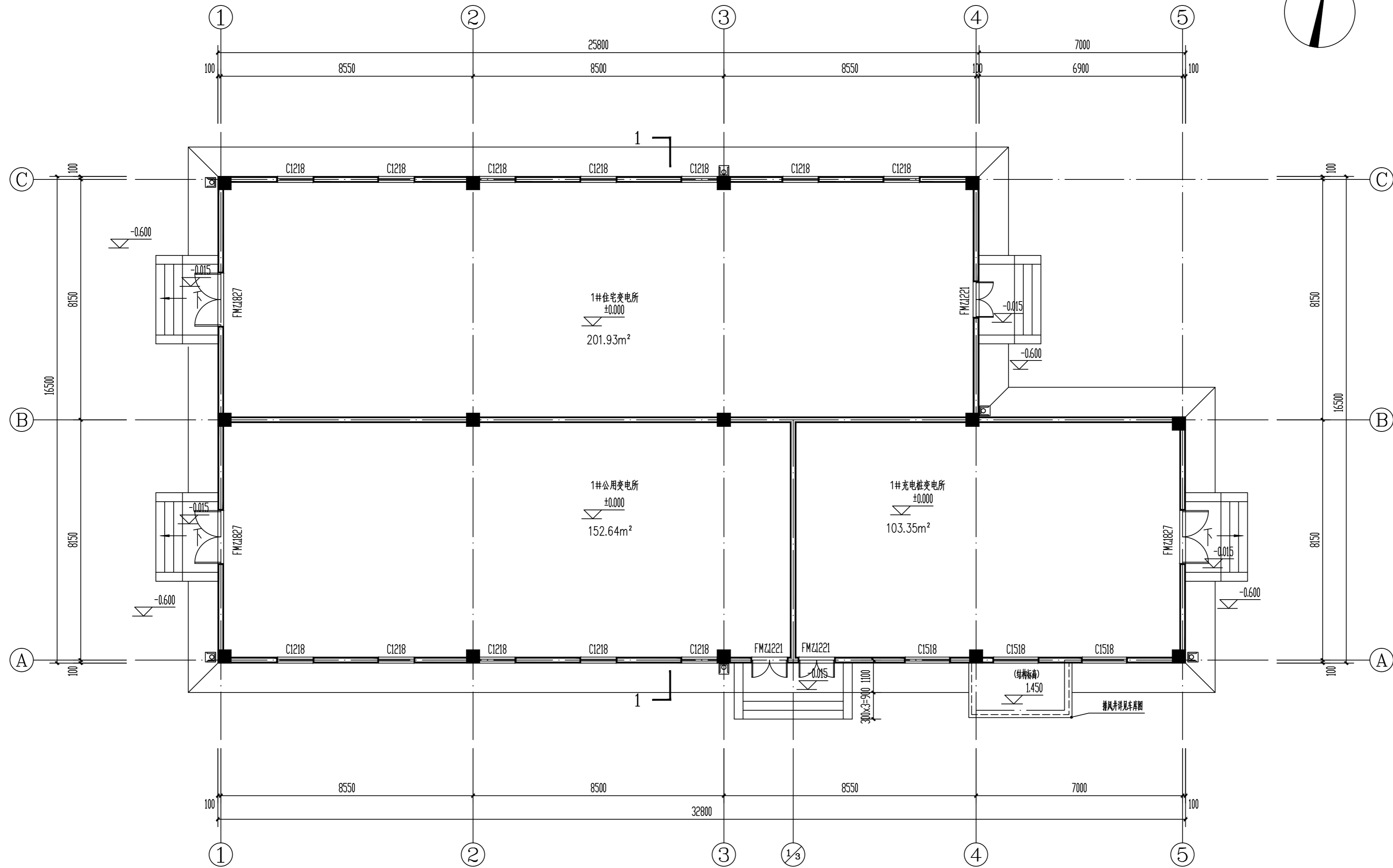
一层平面图 1:100
