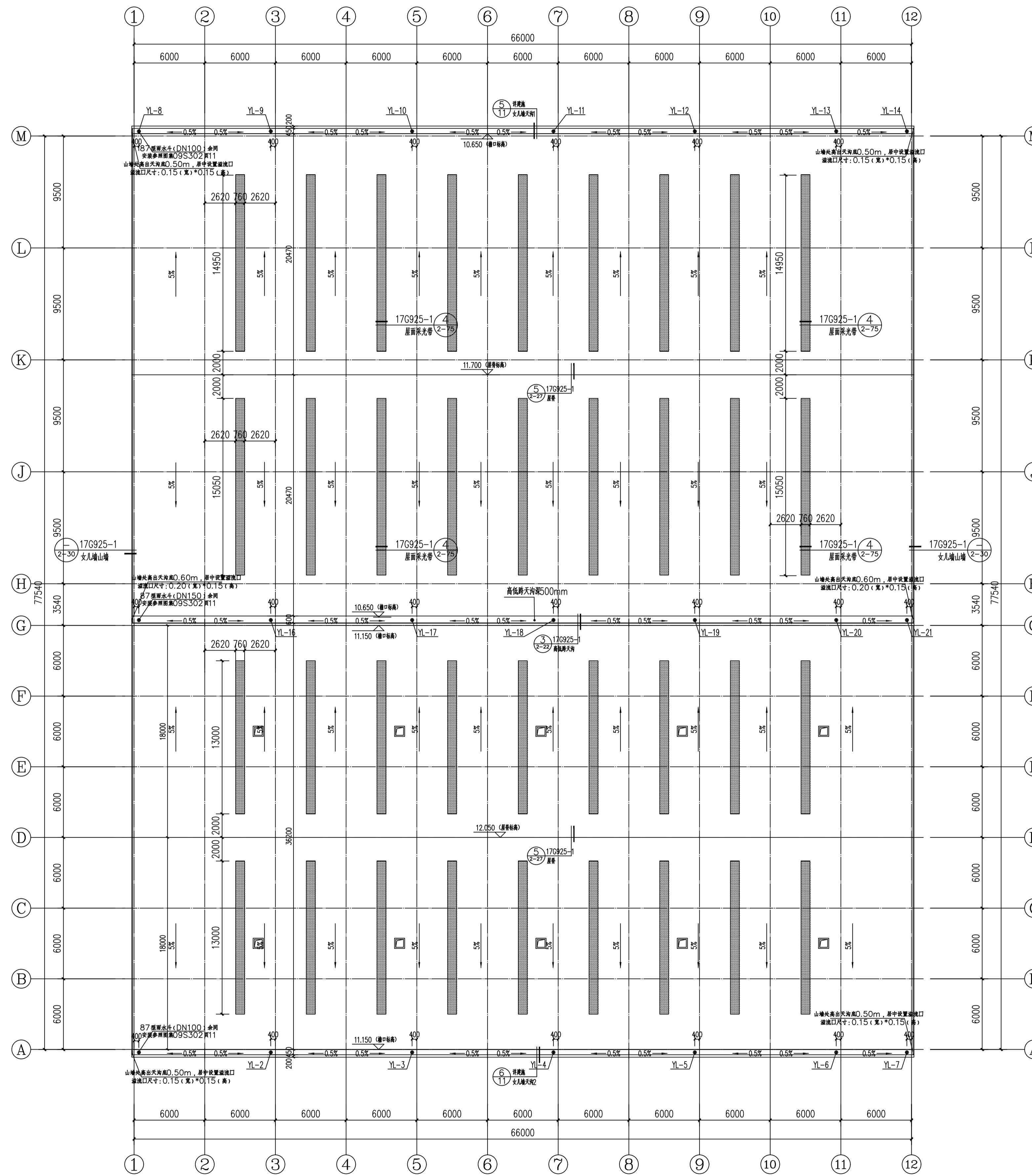
屋顶平面图 1:200
