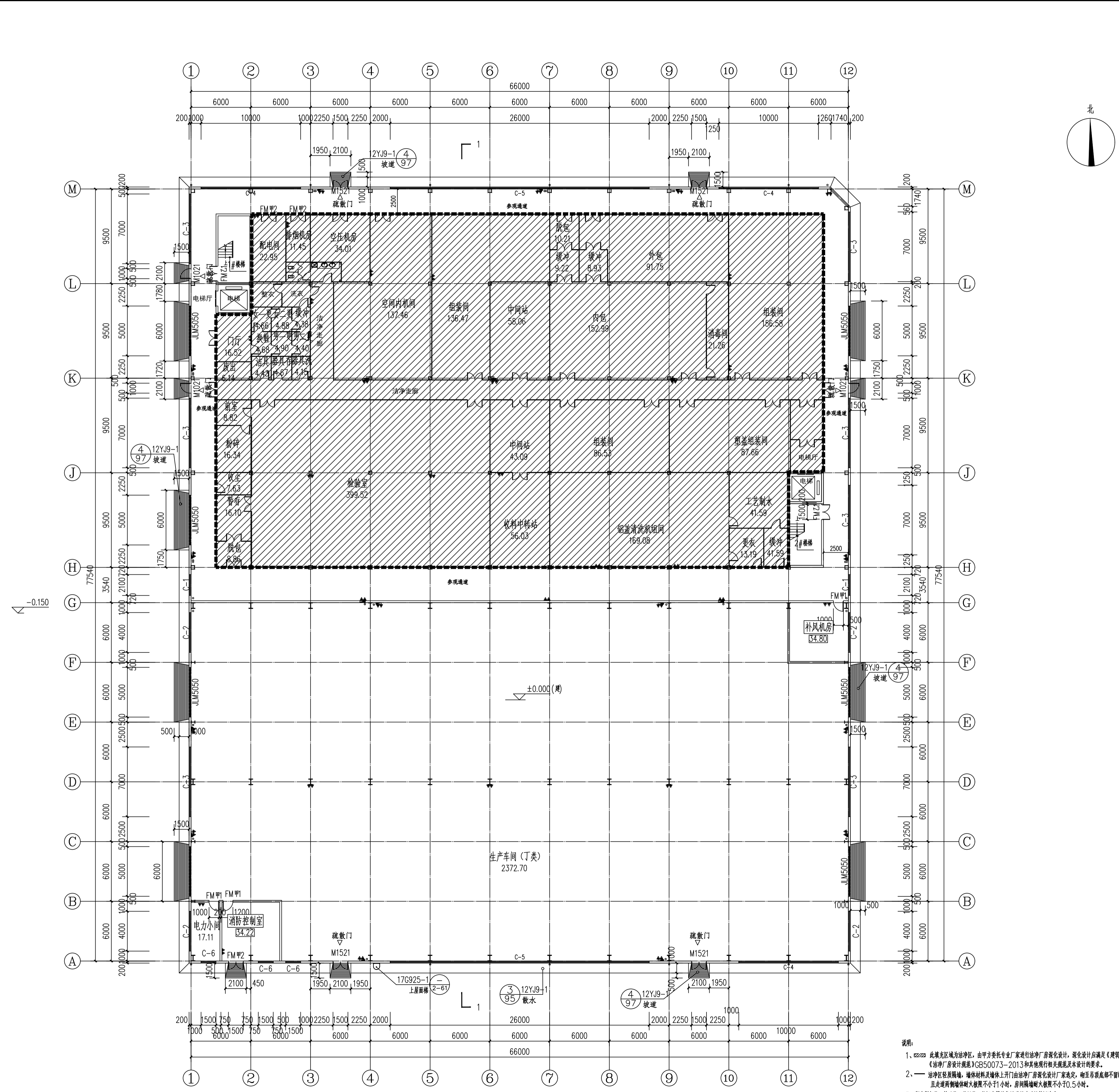
首层平面图 1:200 S=5173.22m²
