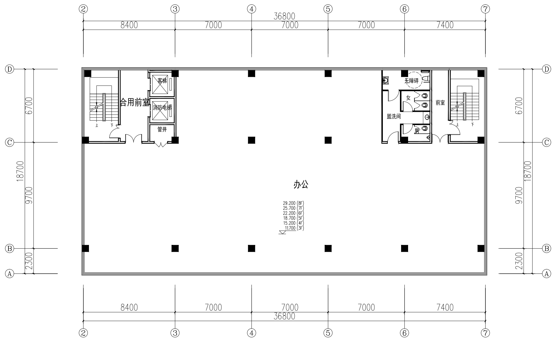
三至八层平面图
