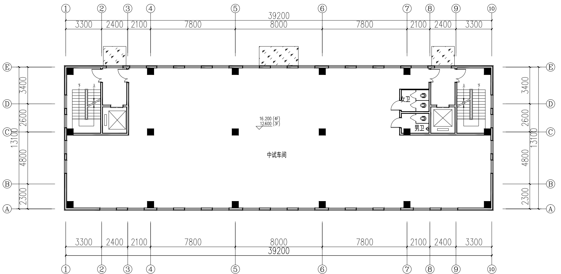
三-四层平面图
