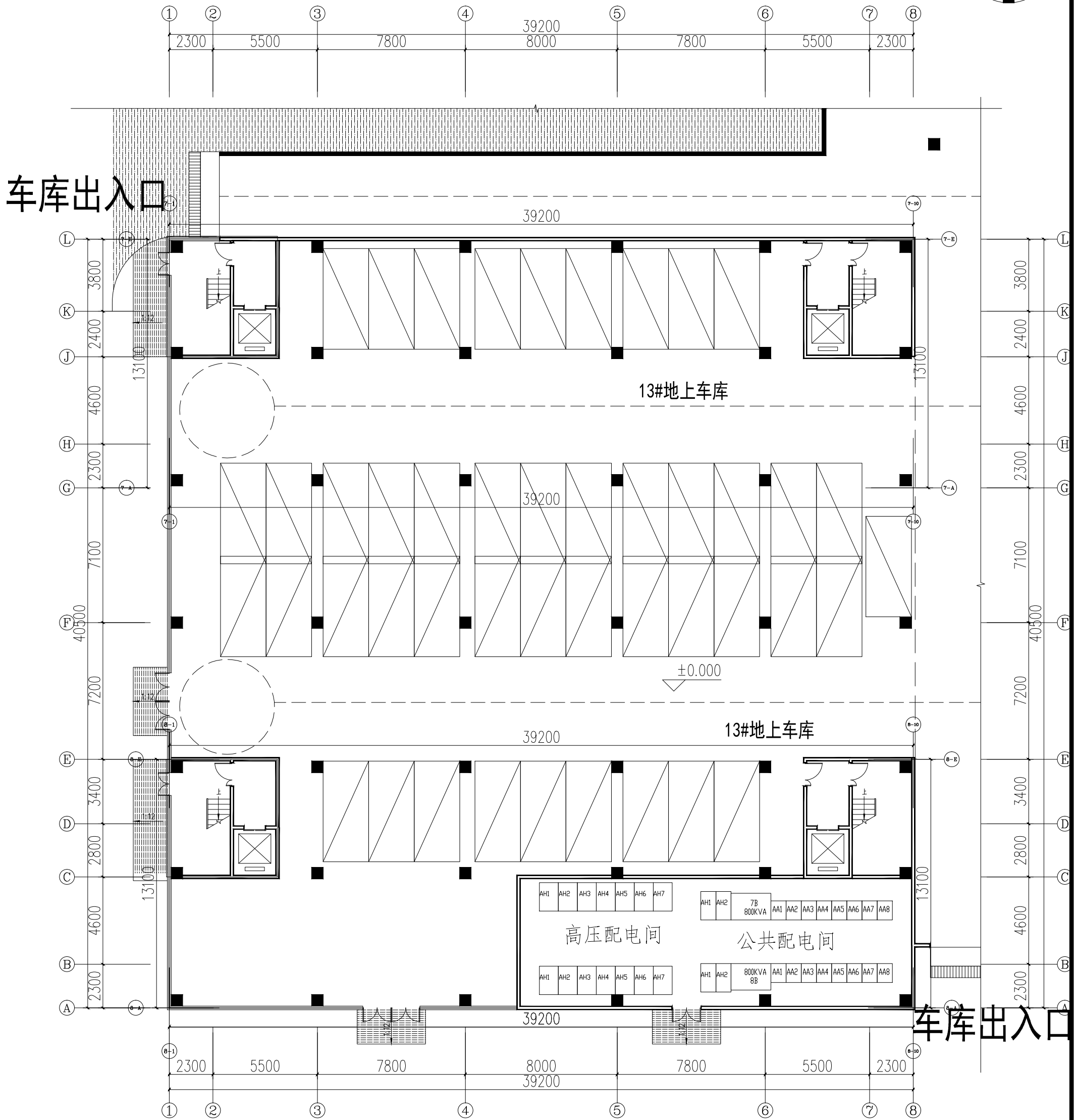
一层平面图
