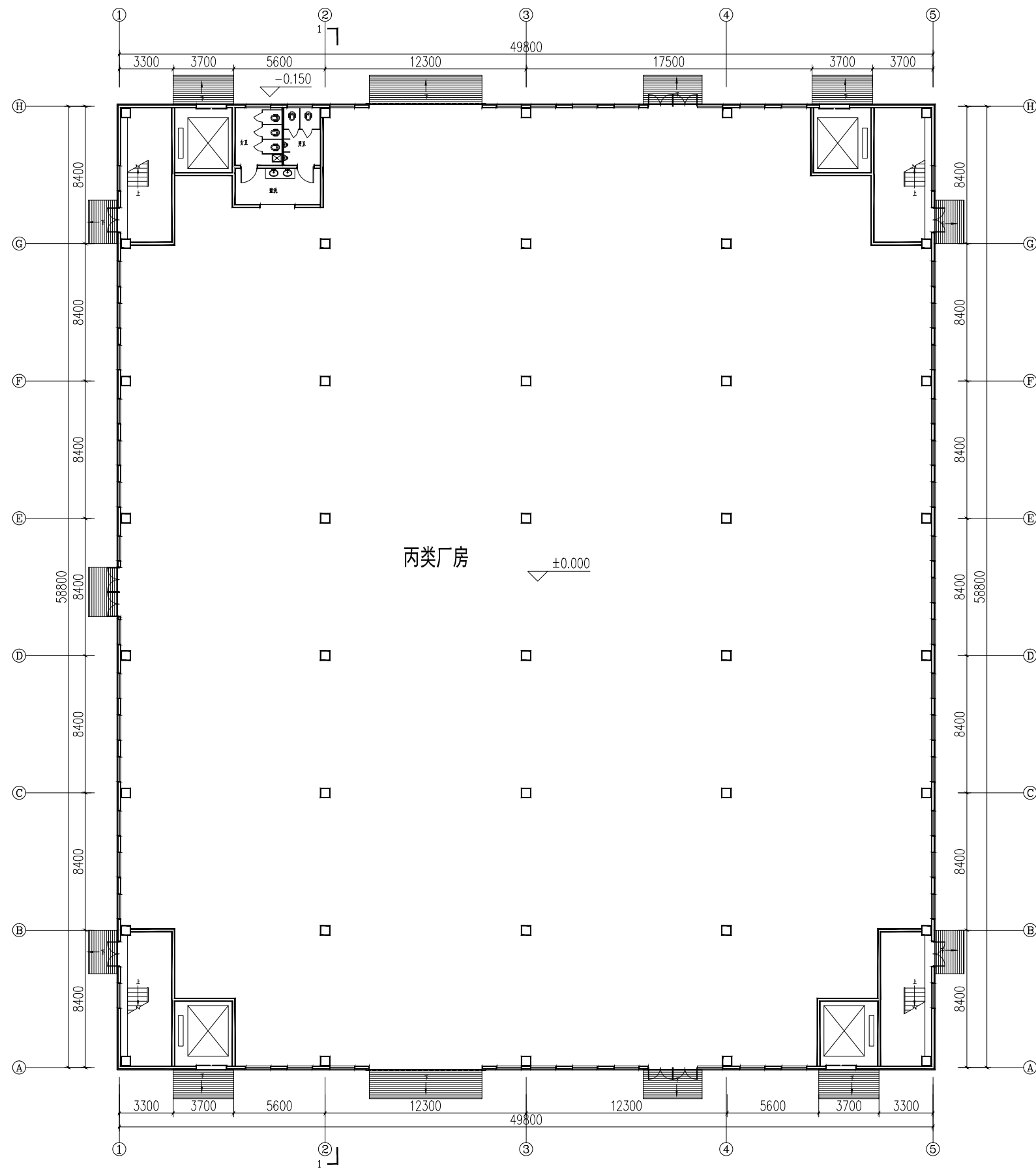
一层平面图
