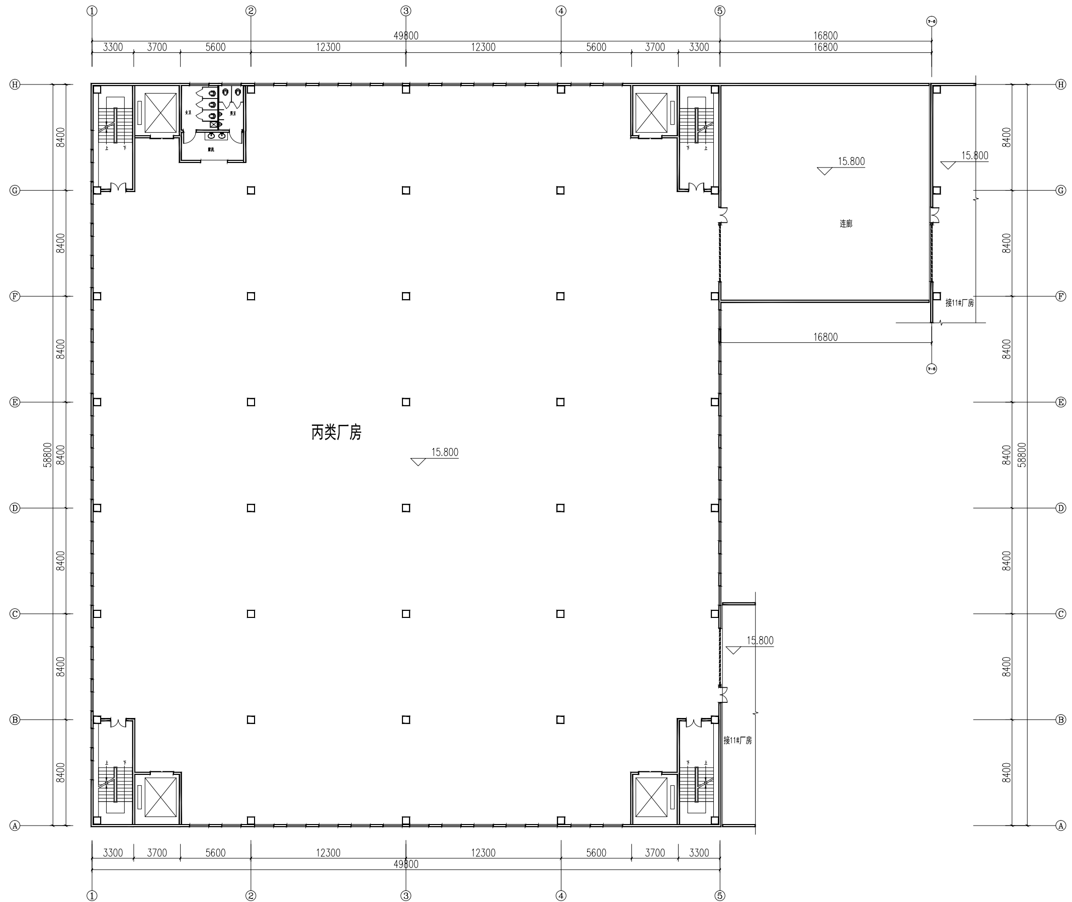
三层平面图
