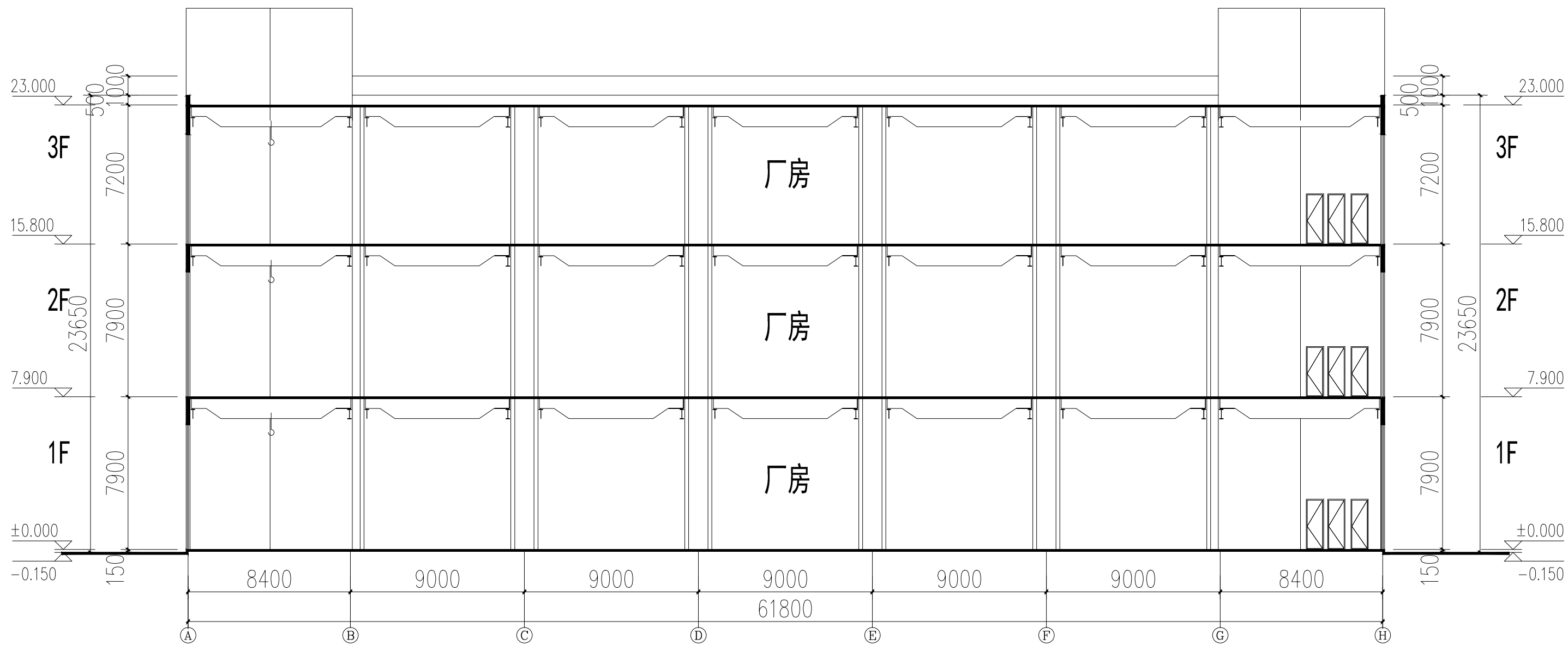
1-1剖面图
