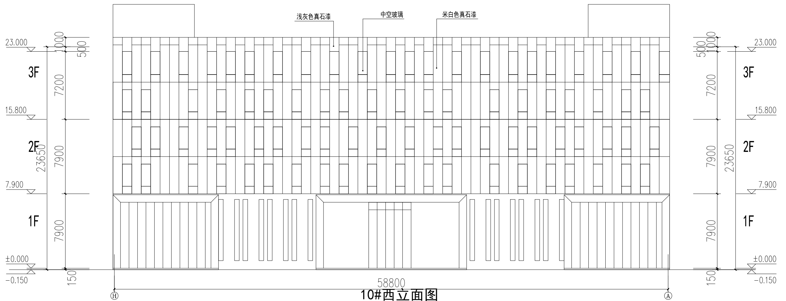
10#南立面图
