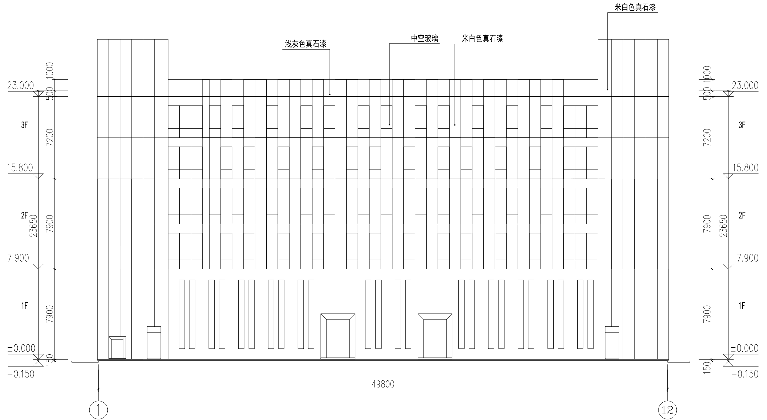
9#南立面图
