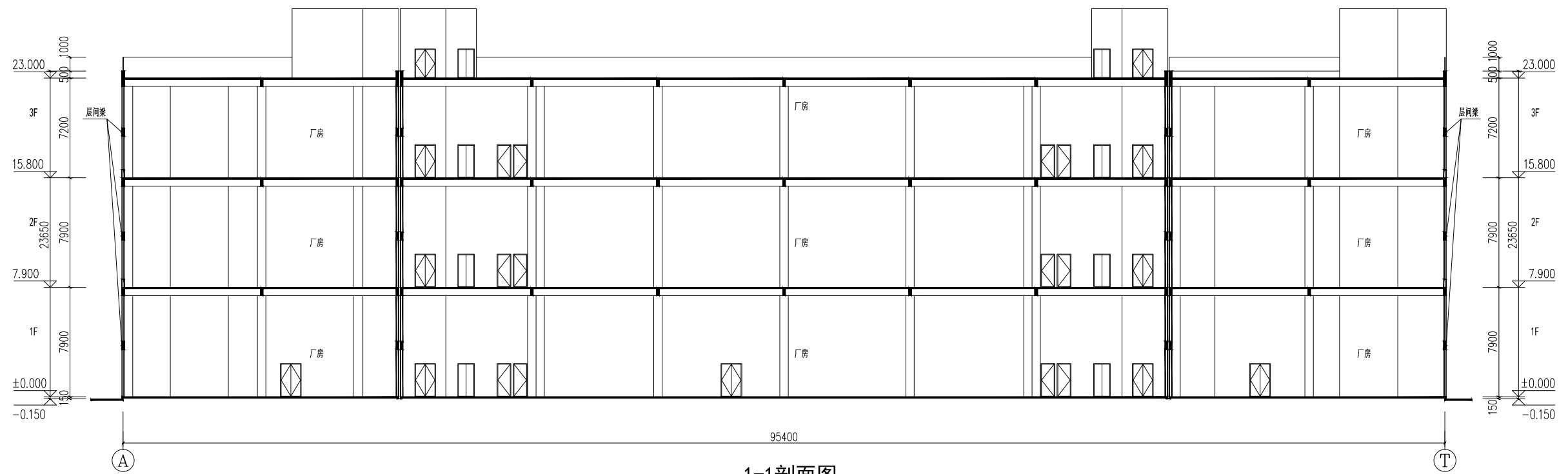
1-1剖面图
