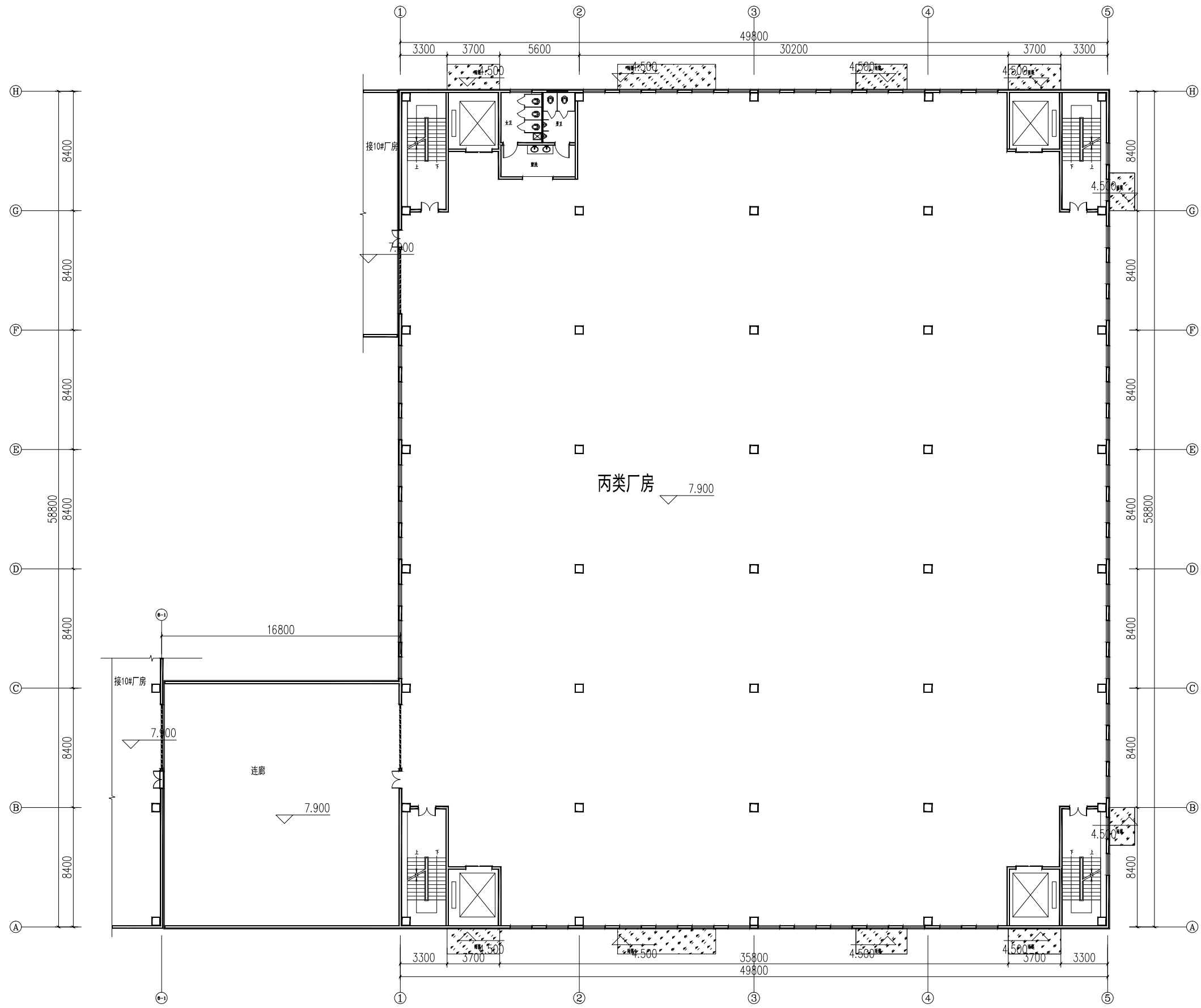
二层平面图
