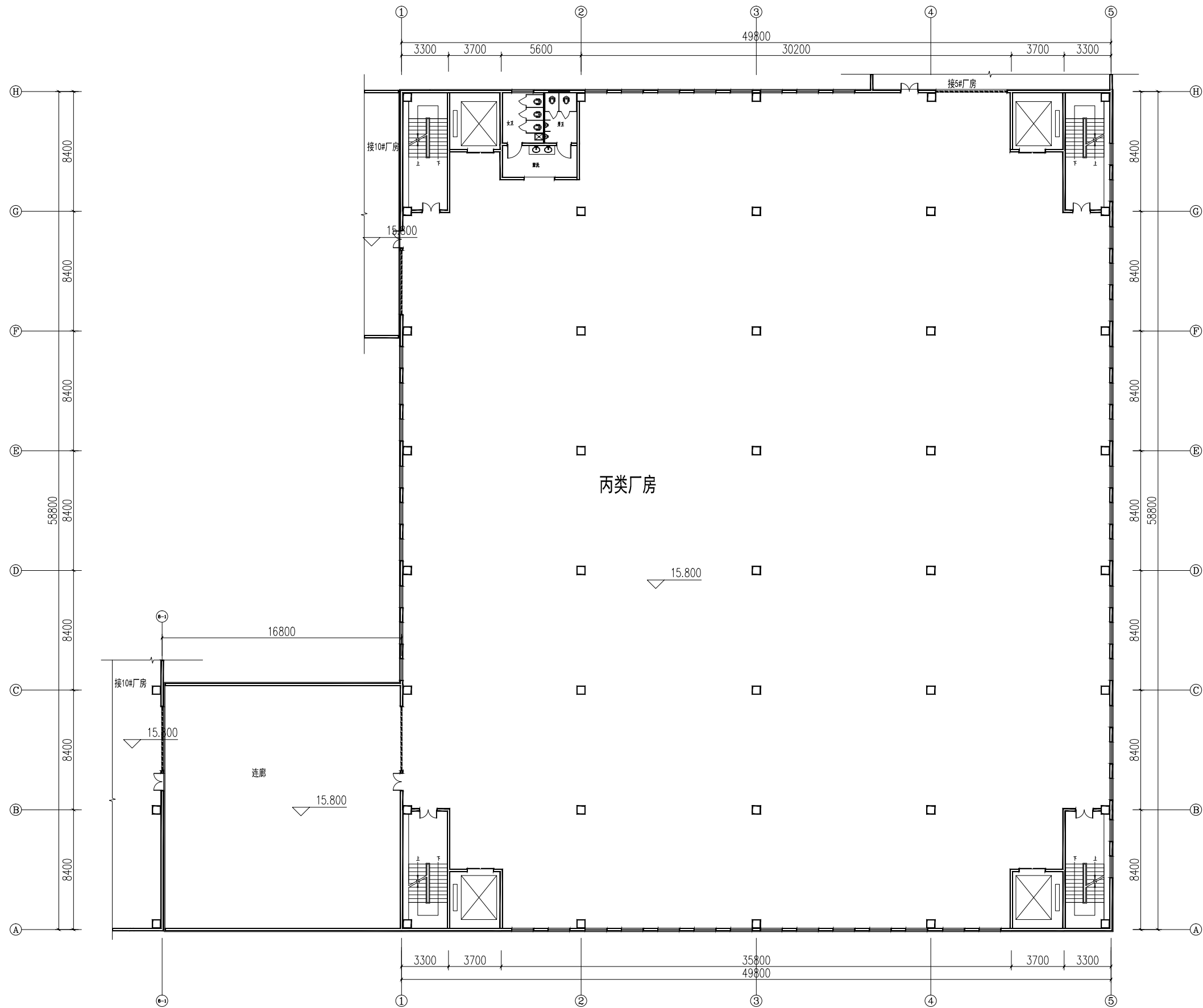
三层平面图
