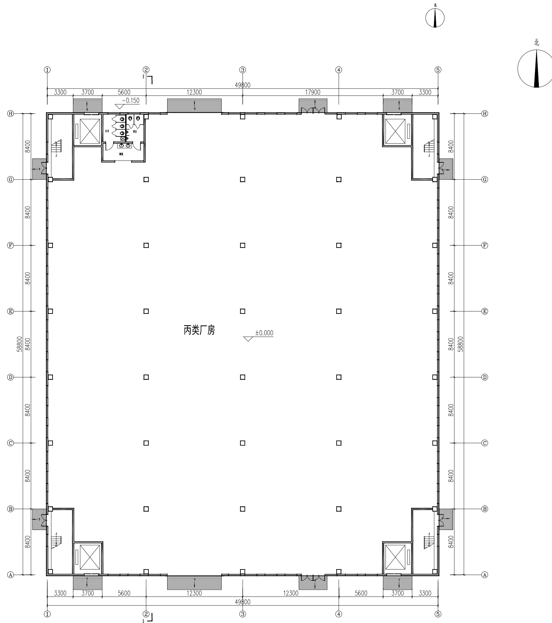
一层平面图
