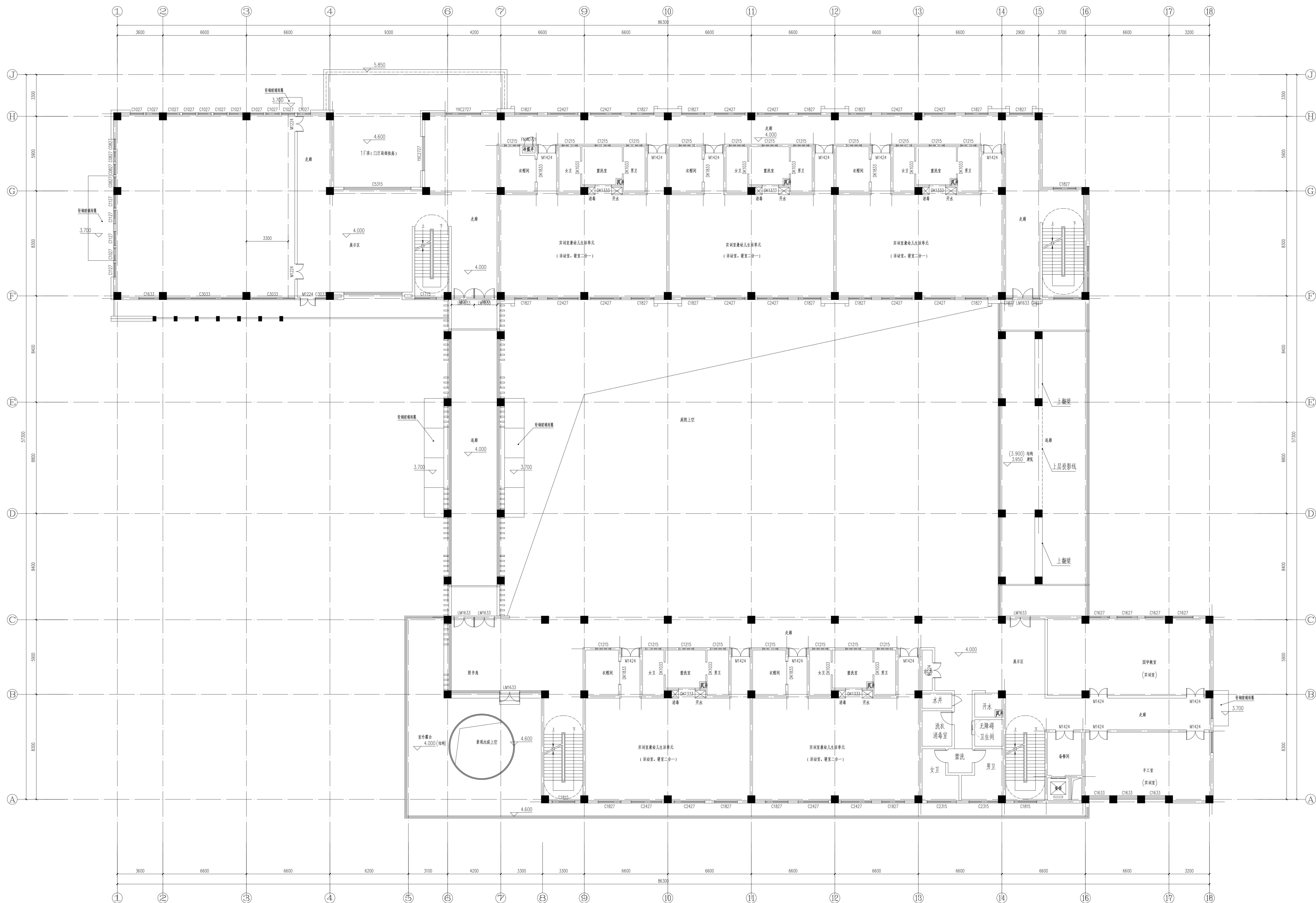
二层平面图 1:100 本层建筑面积2181.28m²
