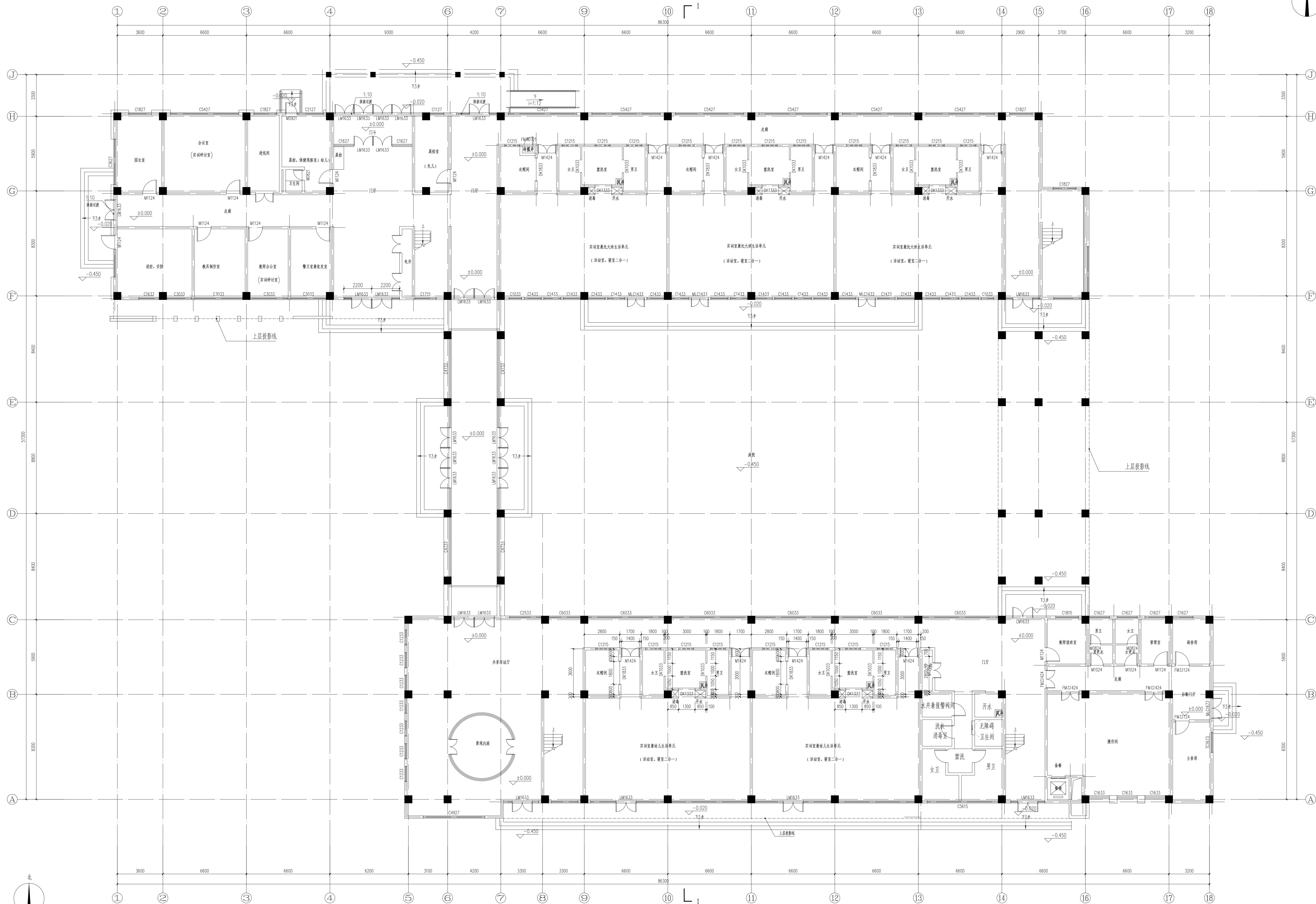
一层平面图 1:100 本层建筑面积2490.94m 2 本工程总建筑面积6463.09m 2
