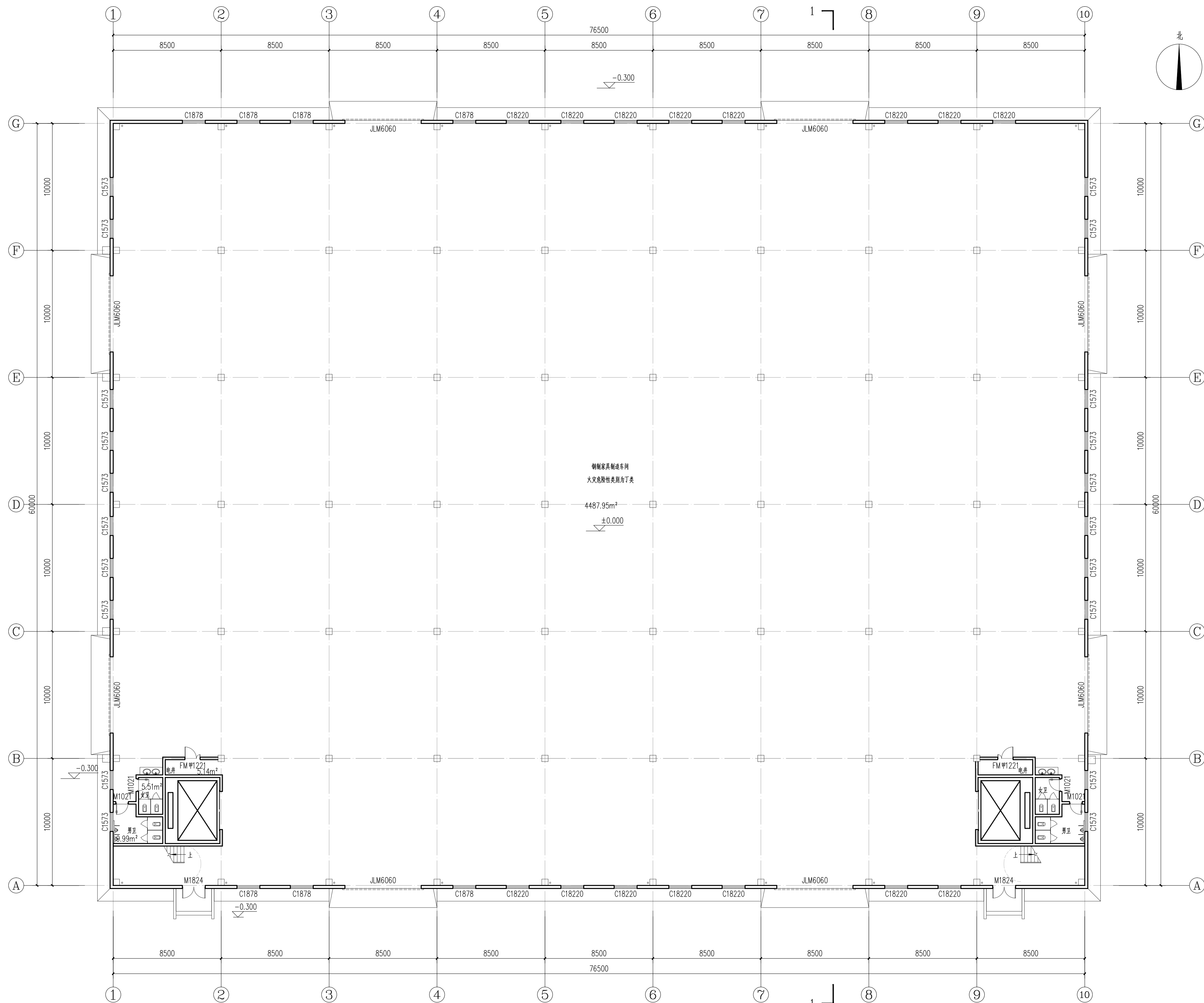
一层平面图 1:150
