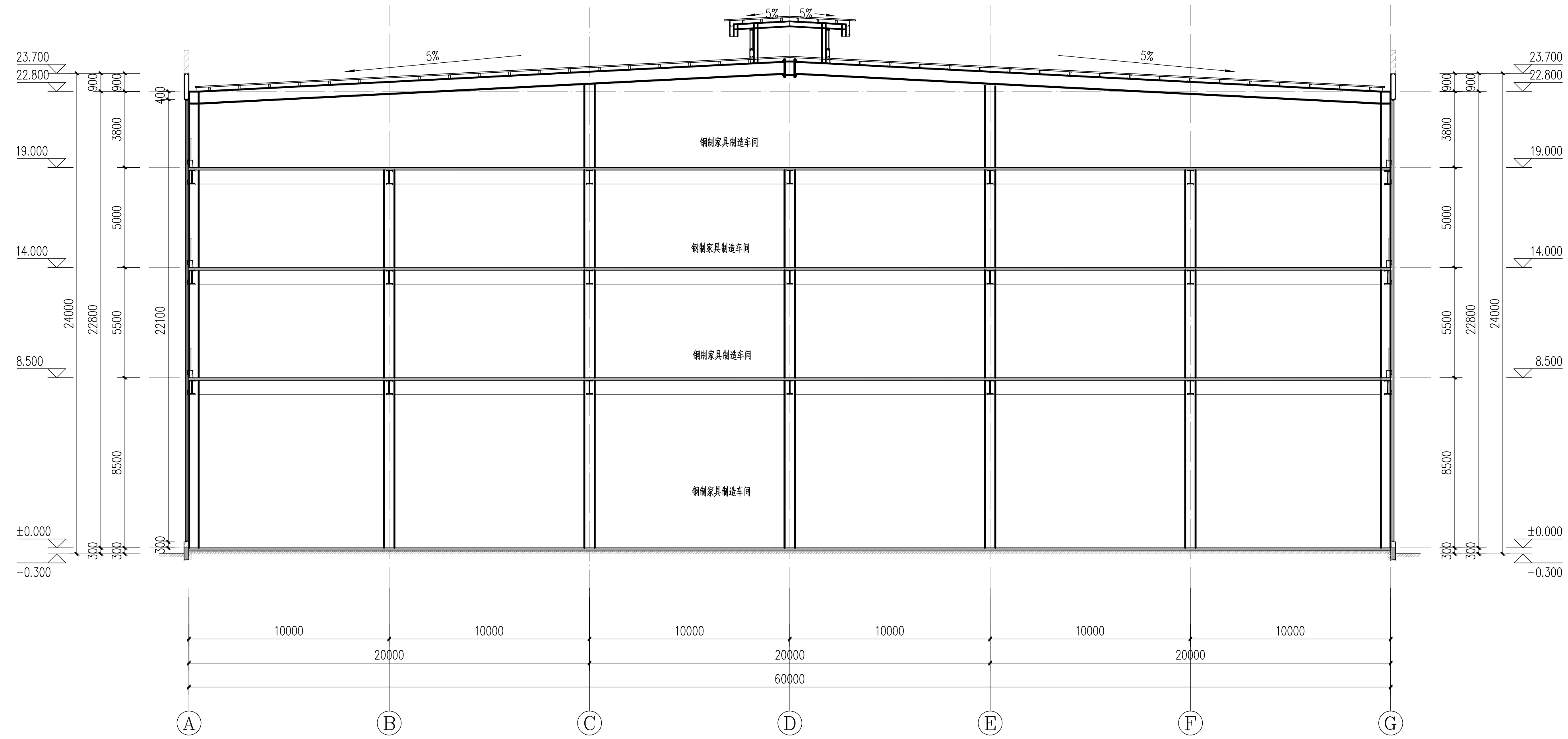
1-1剖面图 1:150
