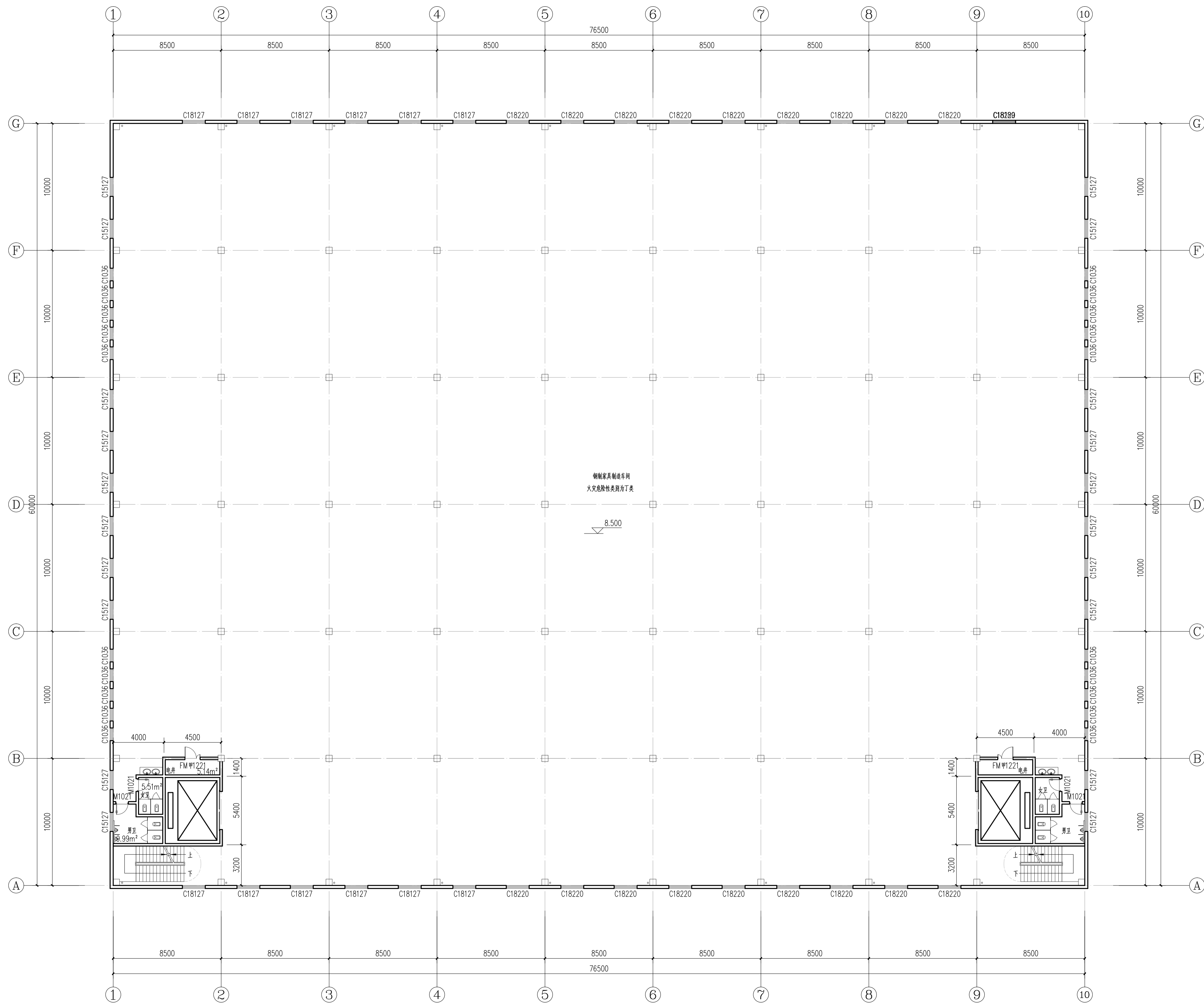
二层平面图 1:150
