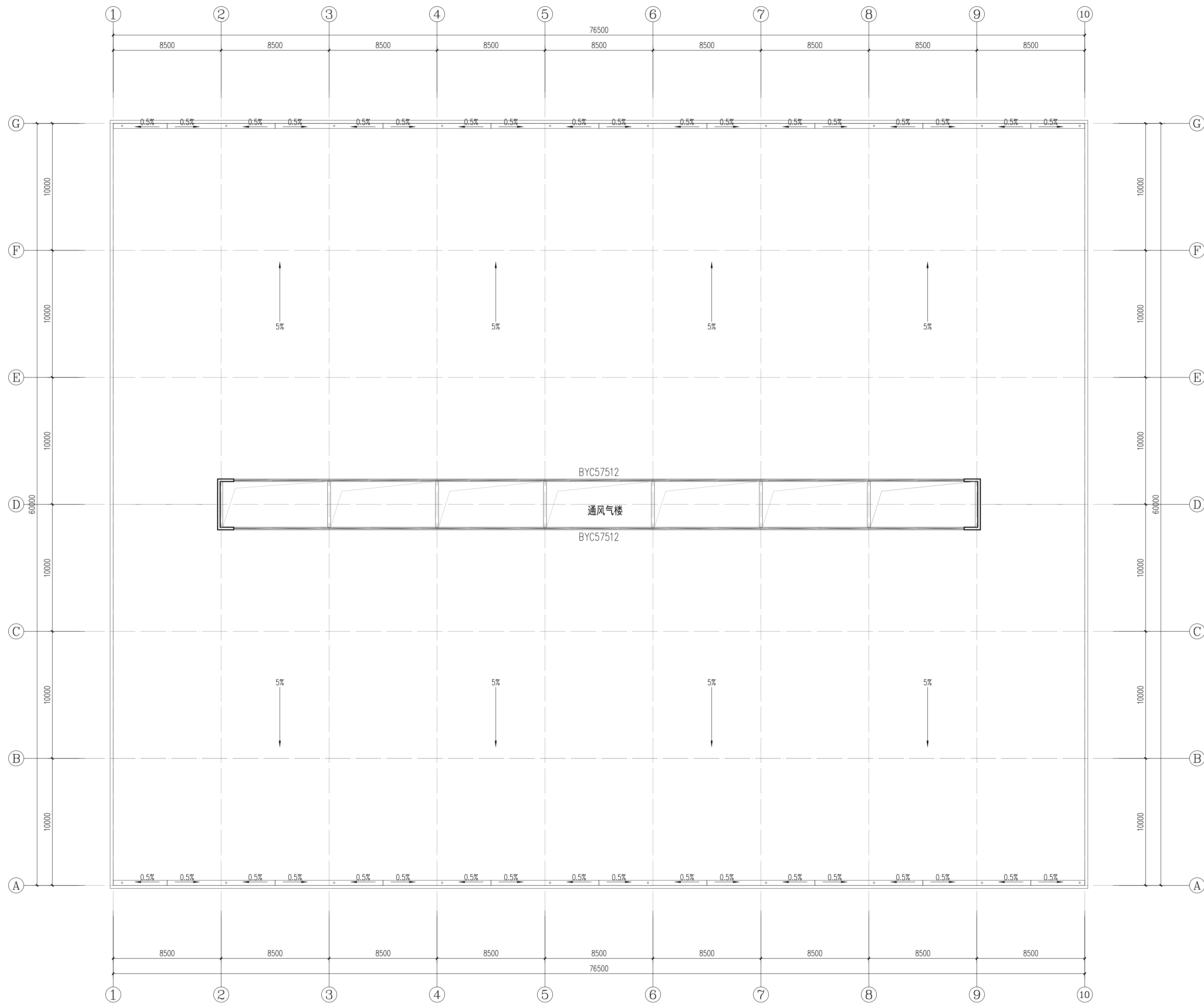
屋顶平面图 1:150
