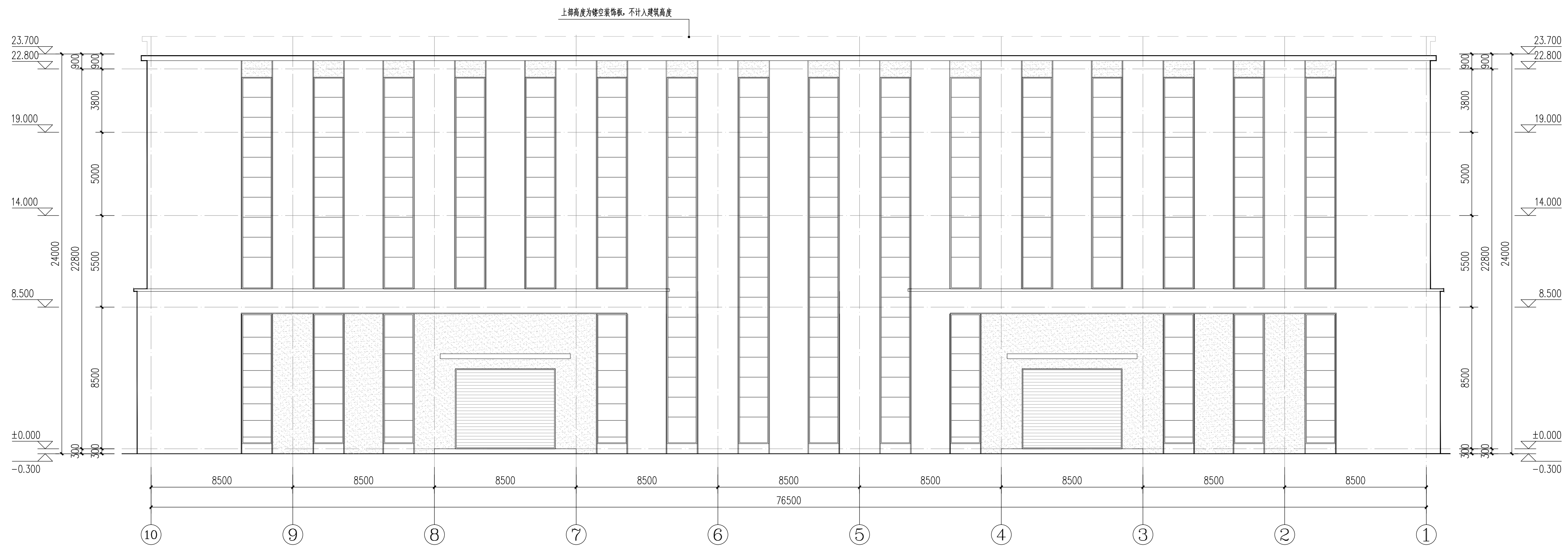
⑩~①轴立面图 1:150
