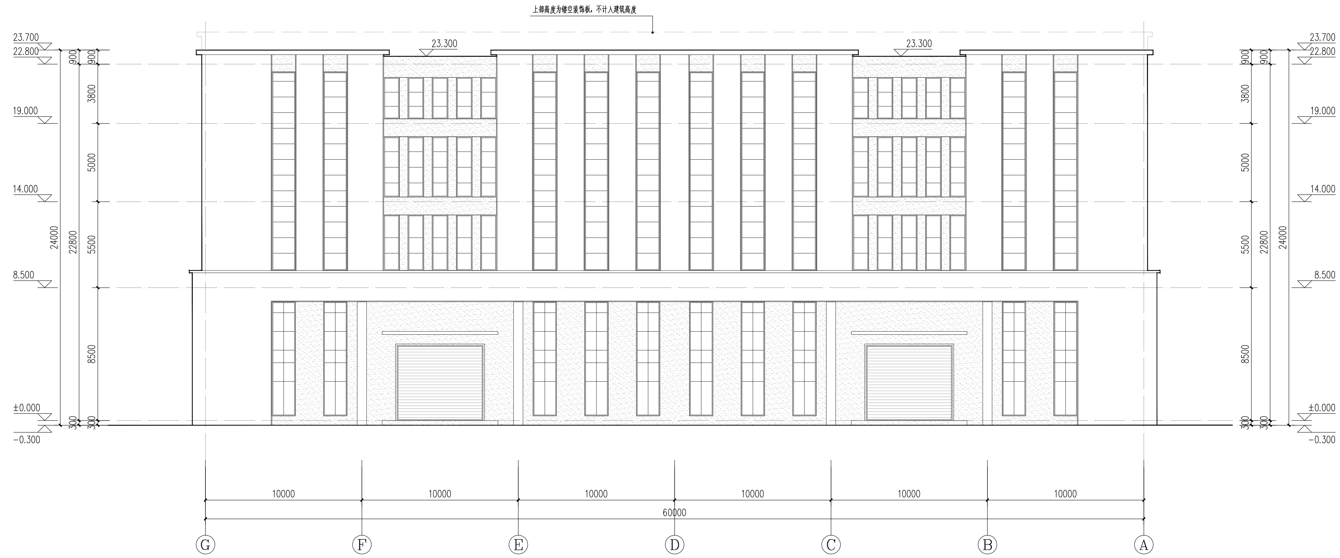
G~A轴立面图 1:150
