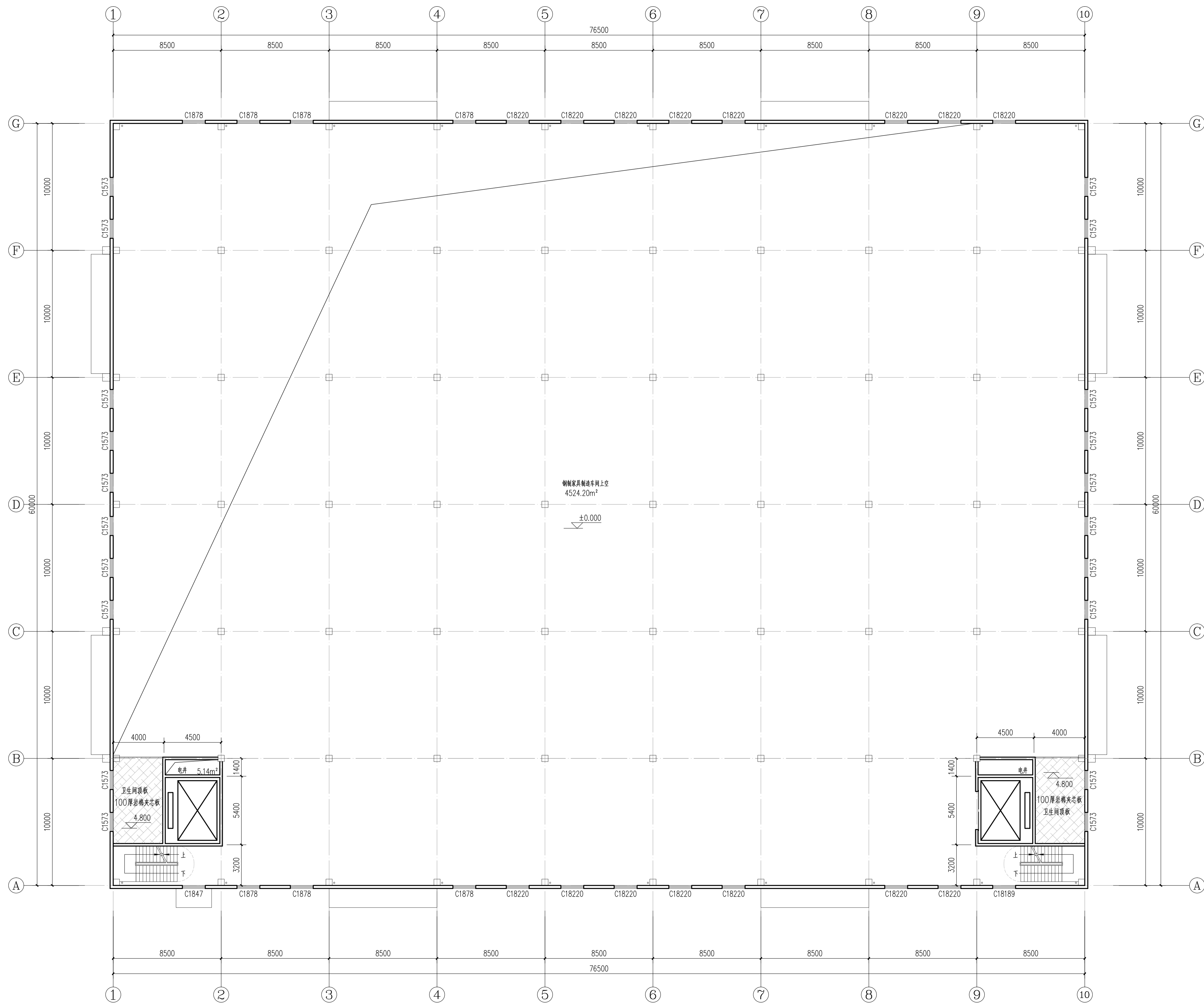
一层上空平面图 1:150
