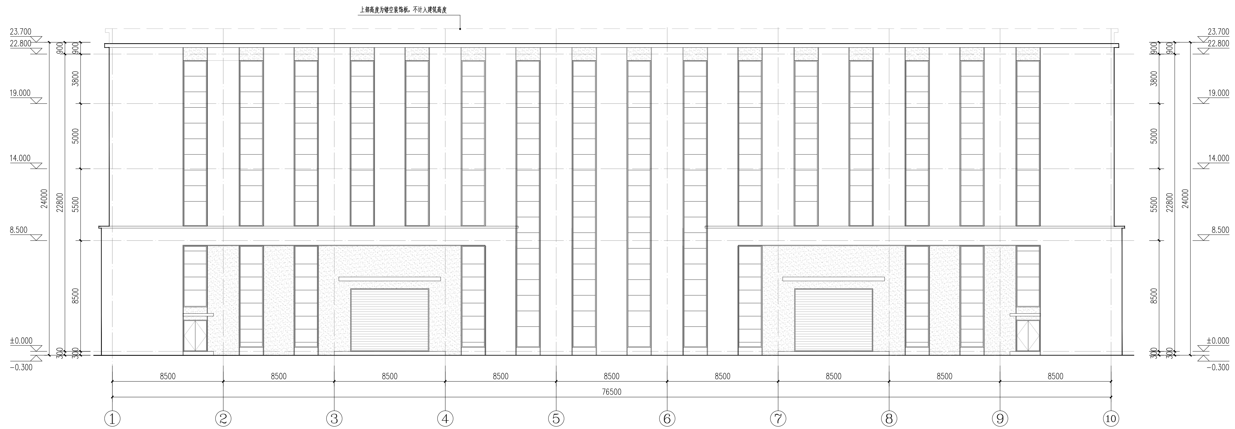
①~⑩轴立面图 1:150
