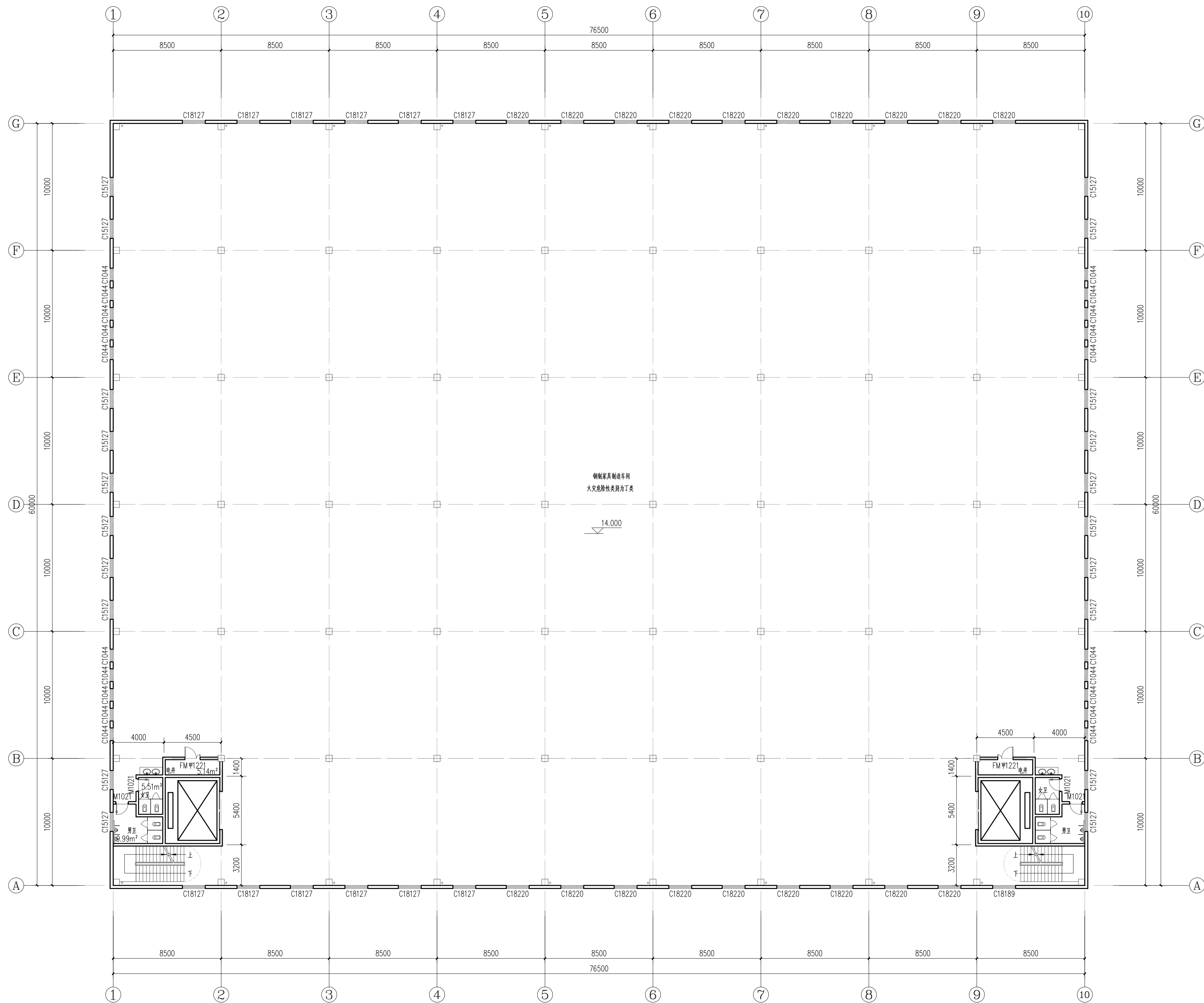
三层平面图 1:150
