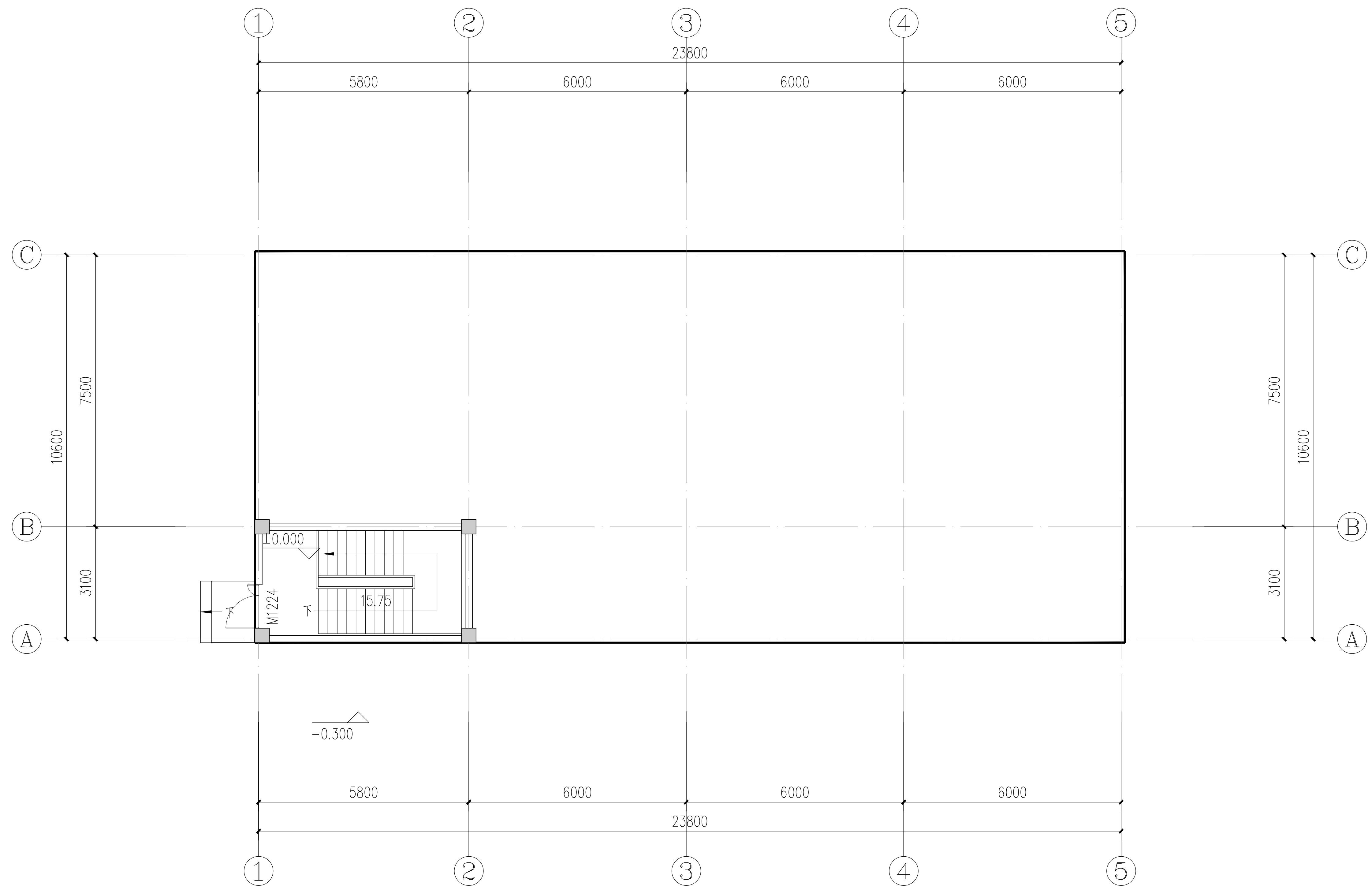
一层楼梯间平面图 1:100 本层建筑面积19.80m 2
