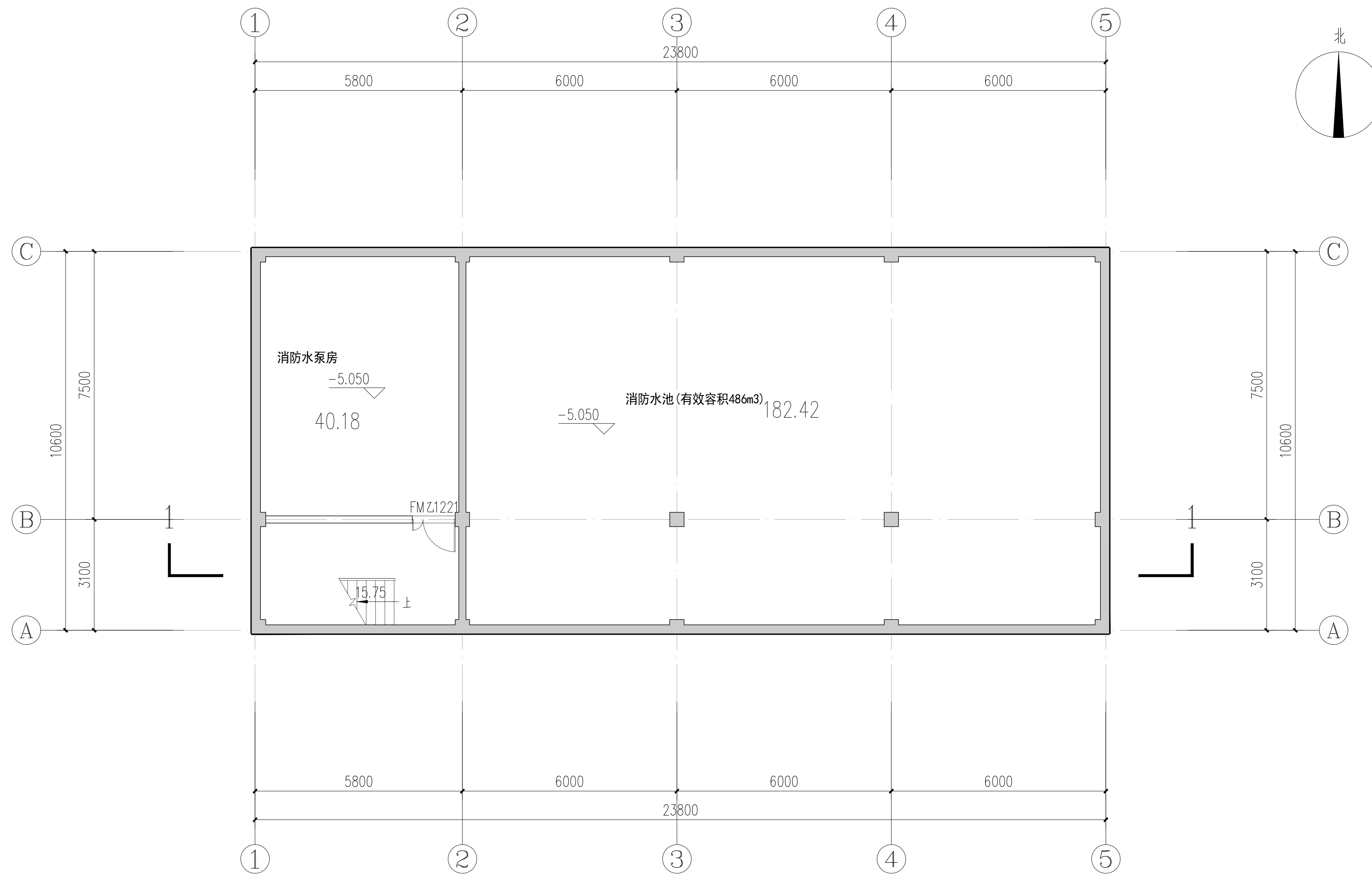
地下消防水池平面图 1:100
