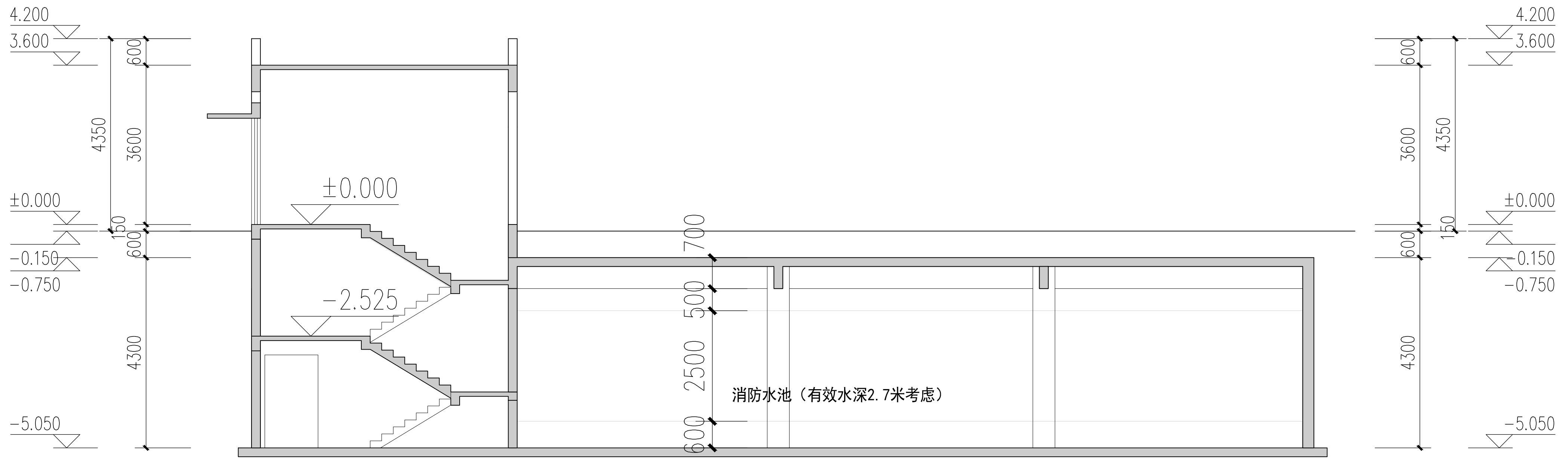
1-1剖面图 1:100
