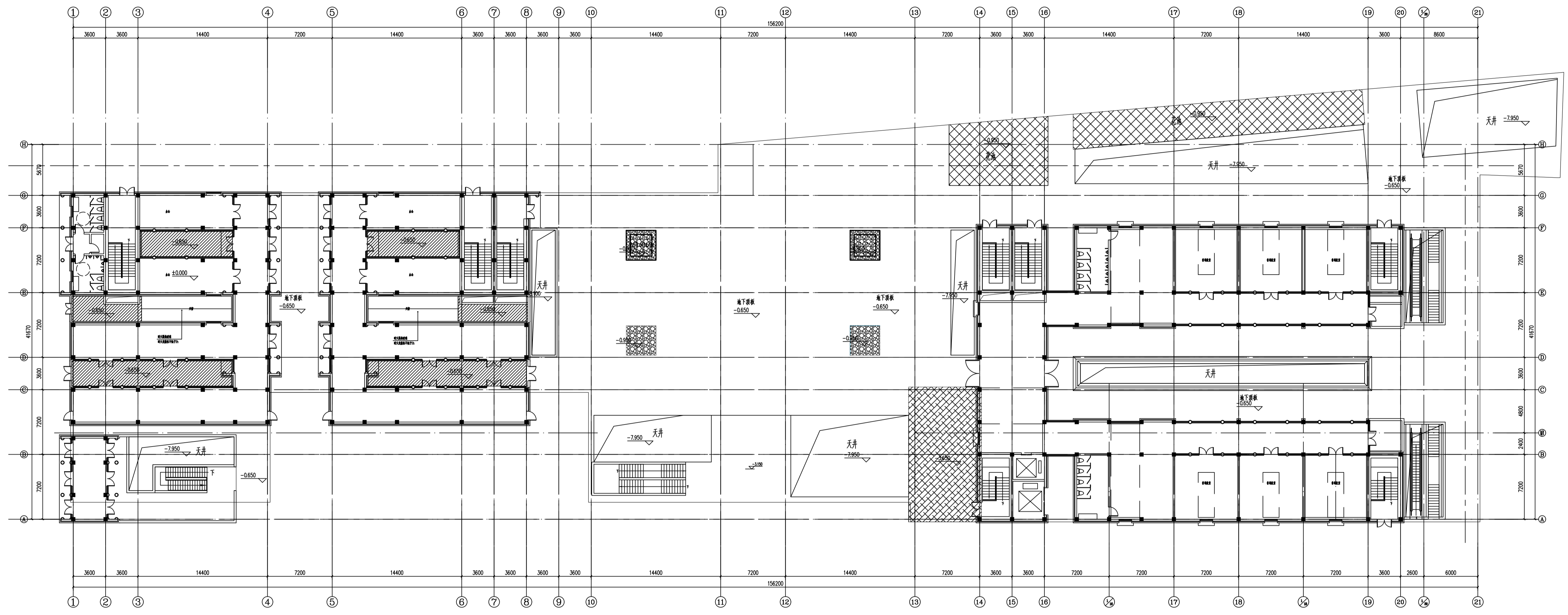
地下车库顶板标高图 1:150
