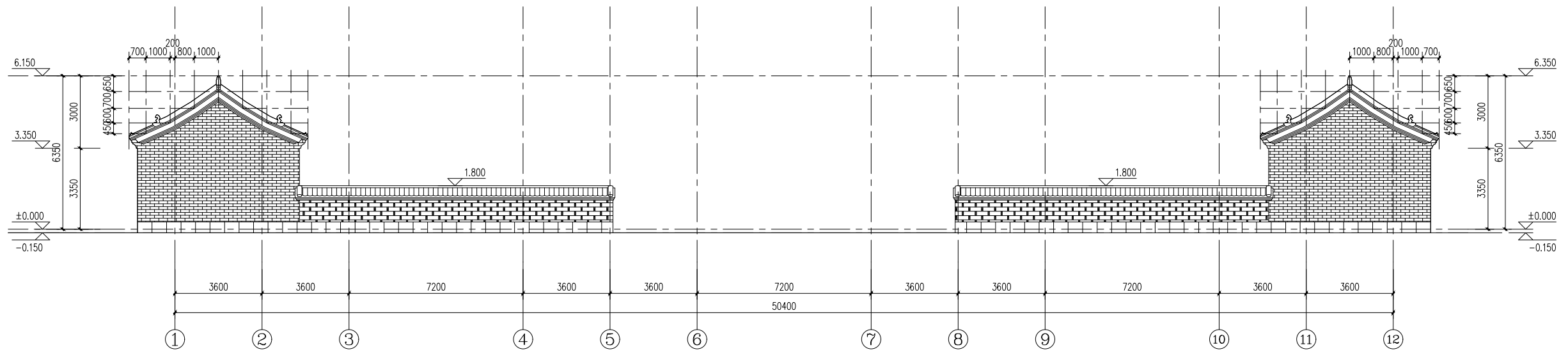
南立面图
