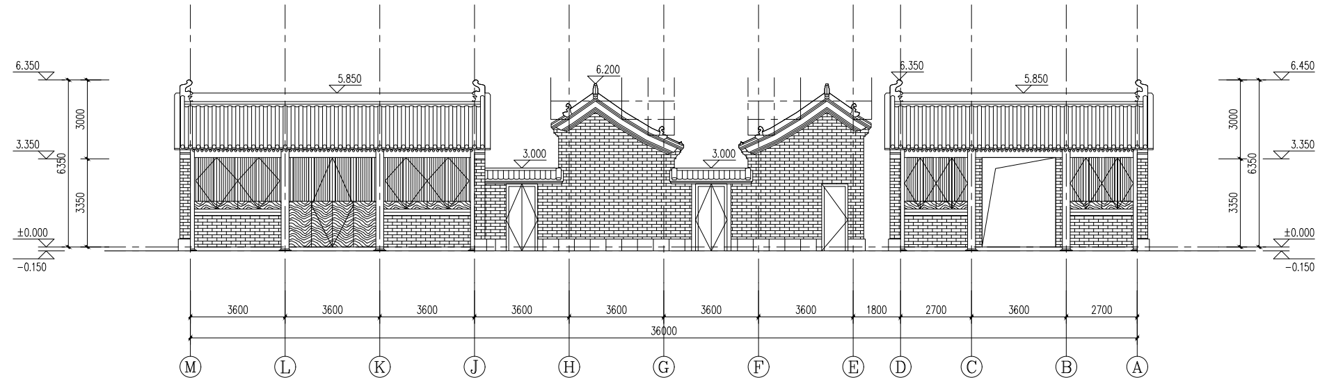
东立面图
