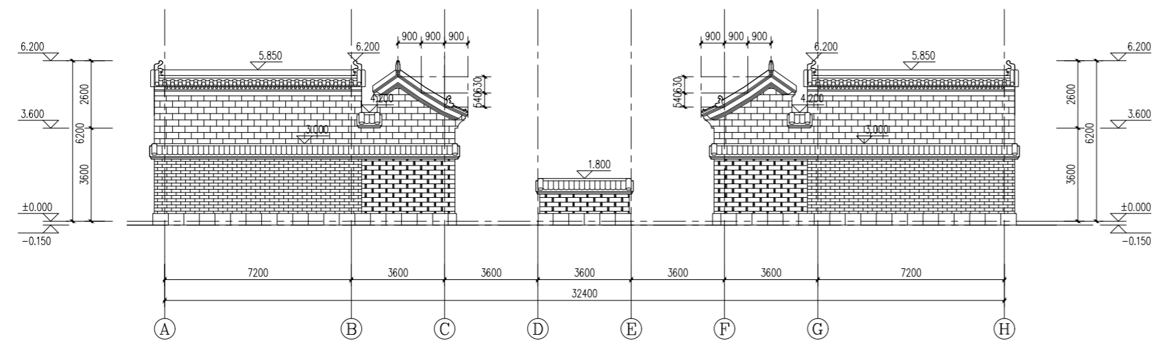
东立面图
