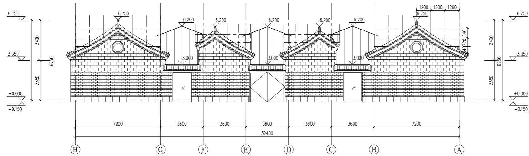
西立面图
