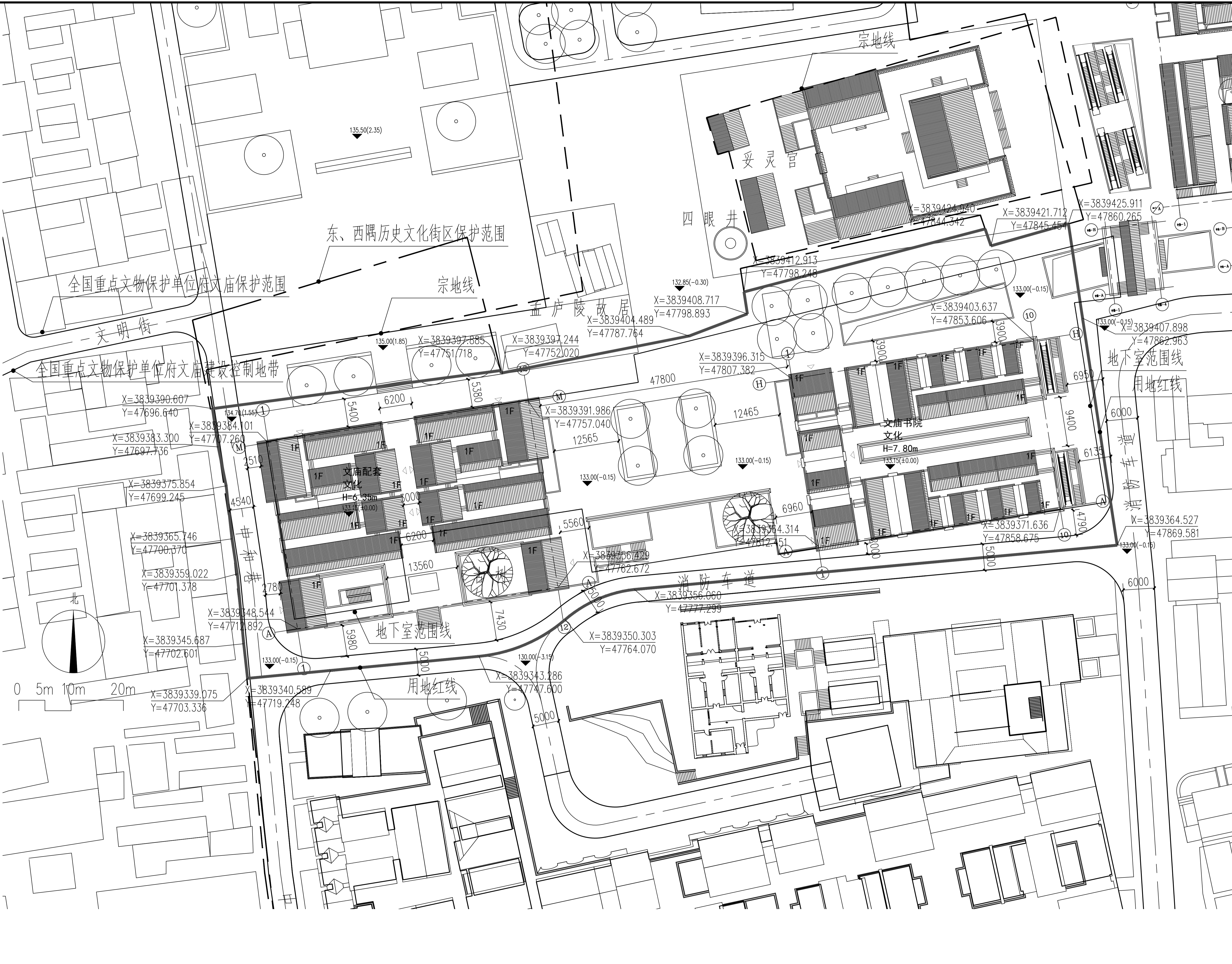
总平面图
