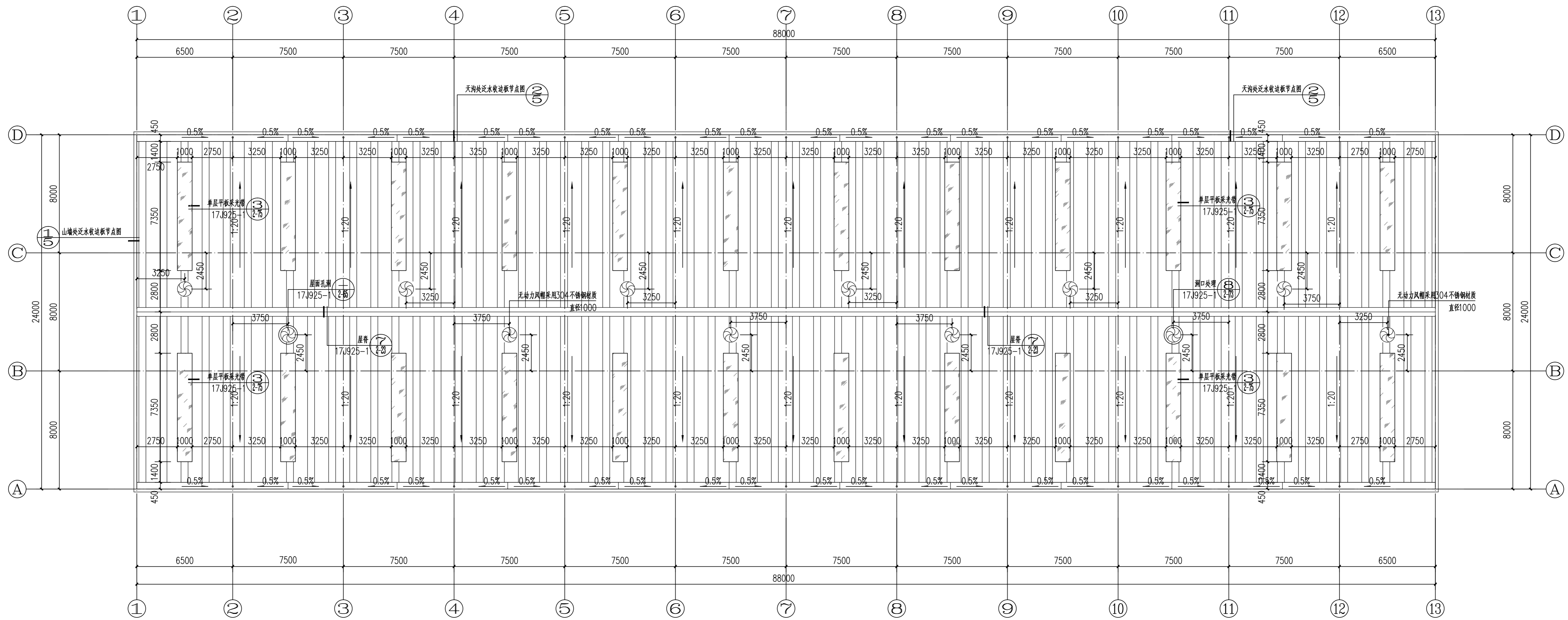
屋顶平面图 1:150
