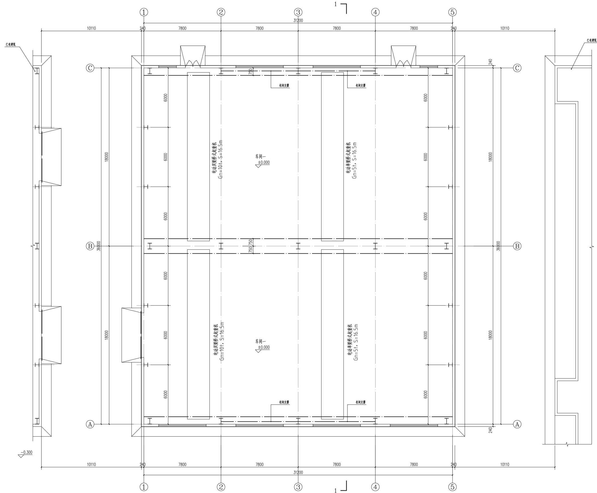
±0.000平面图 1:100
