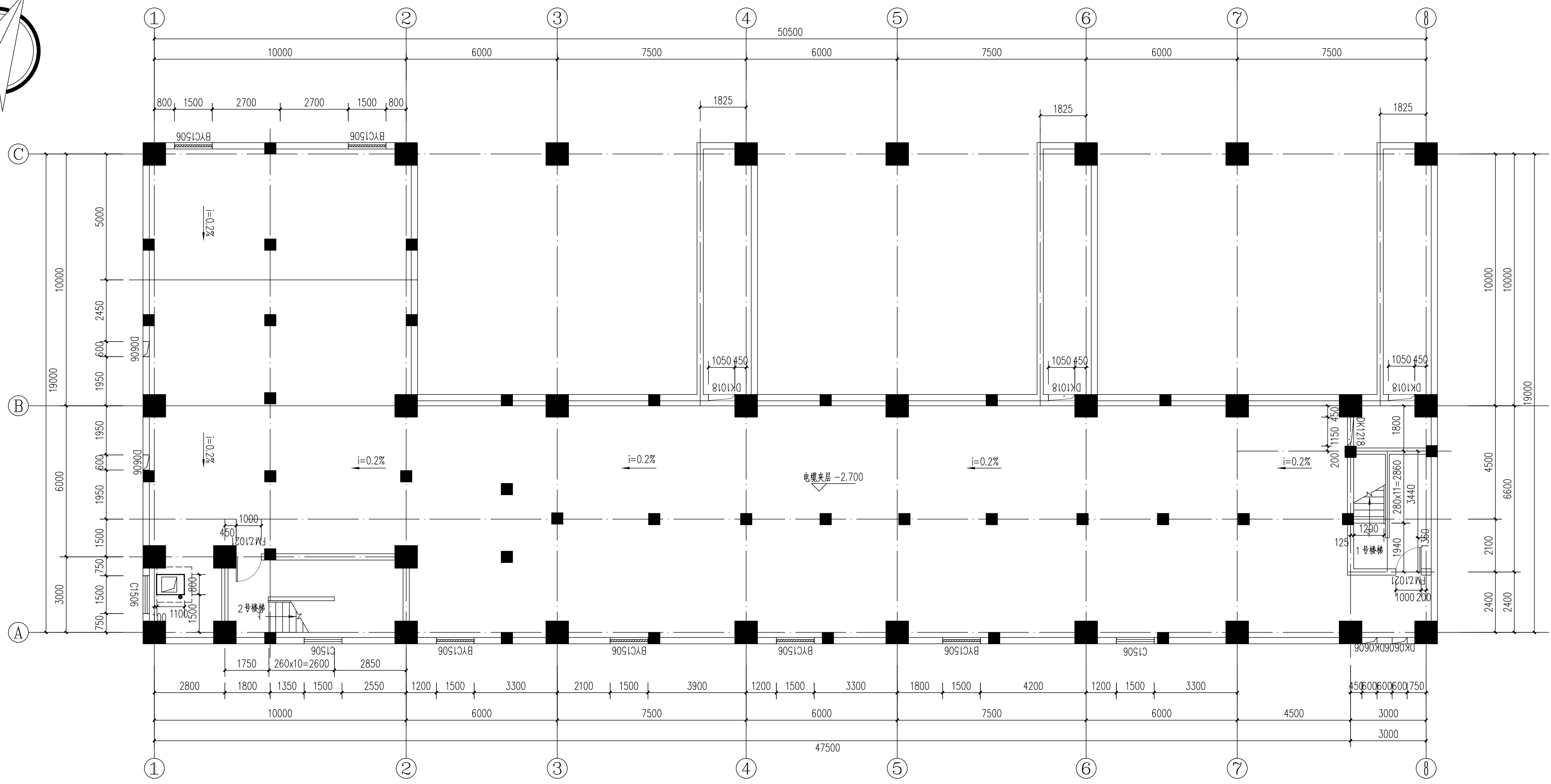
电缆夹层平面图 1:100
