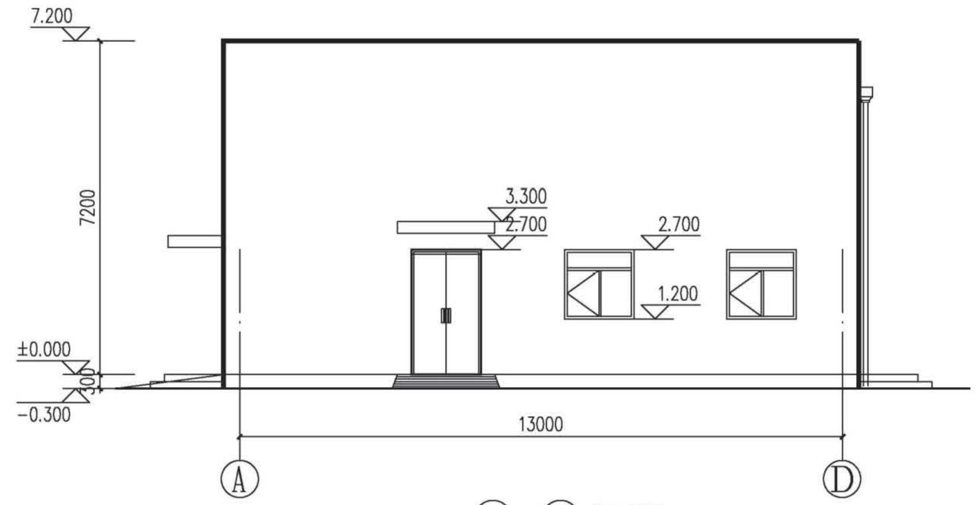
A - D 轴立面图 1:100
