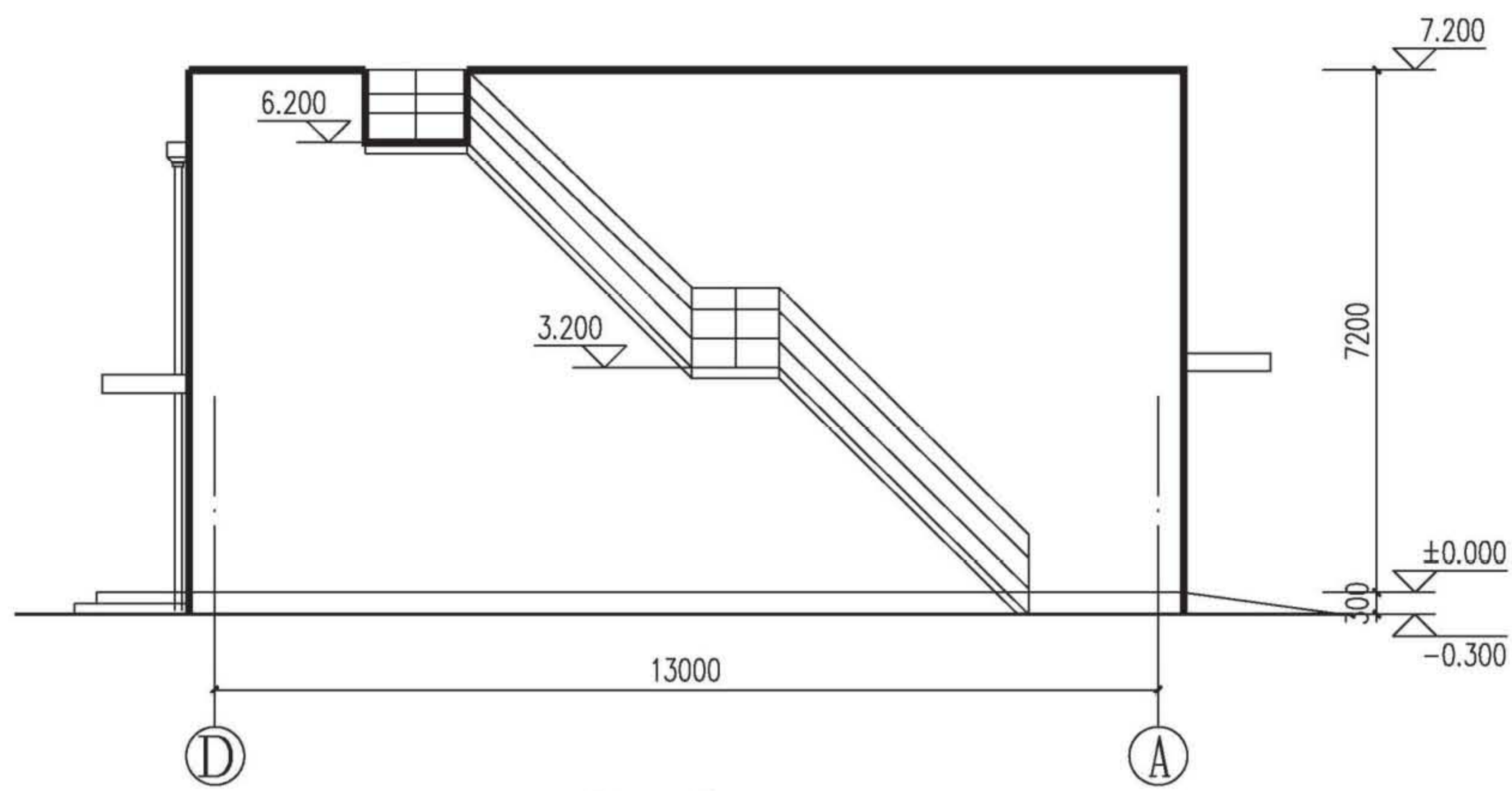
D - A 轴立面图 1:100
