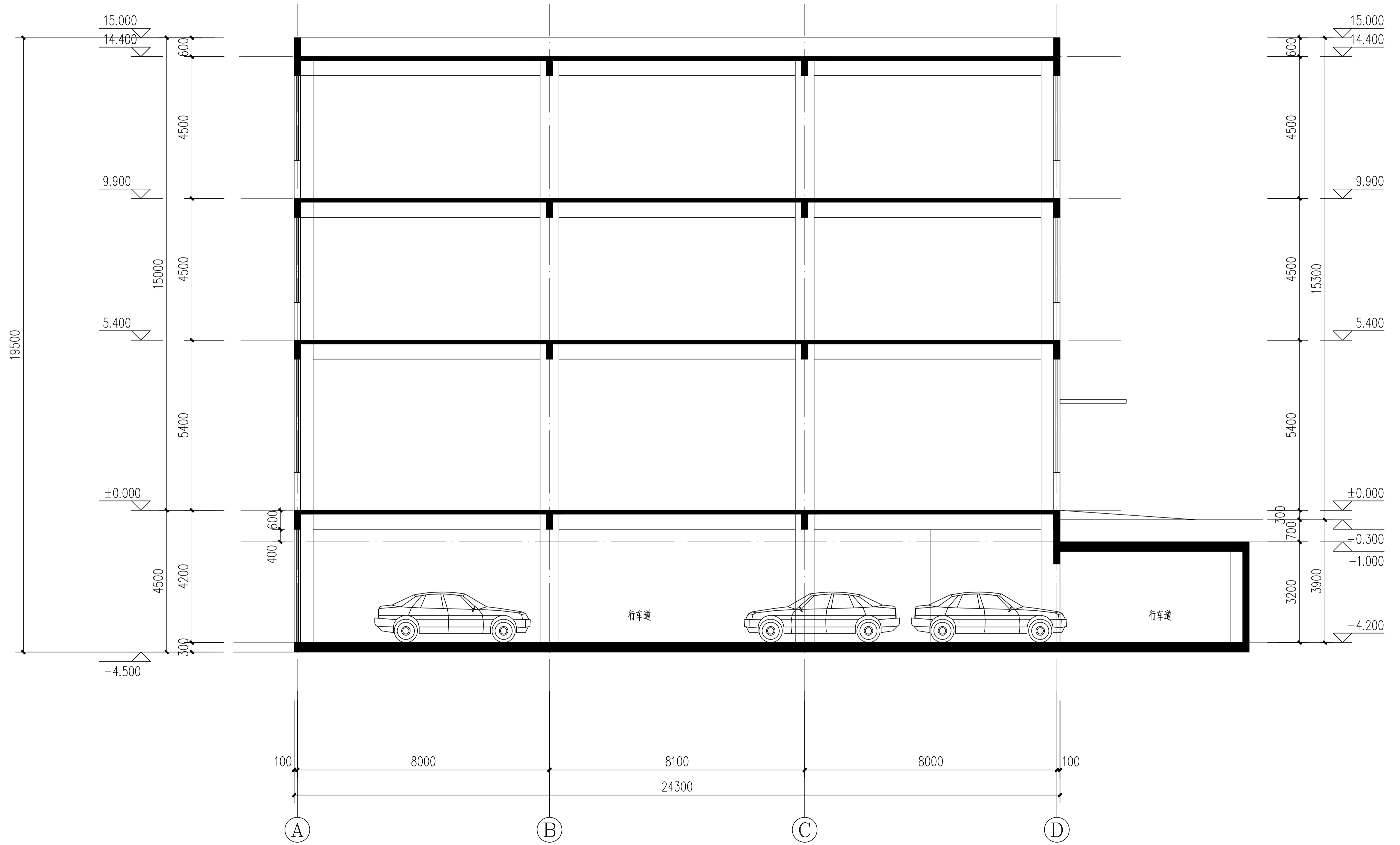
1-1剖面图 1:100
