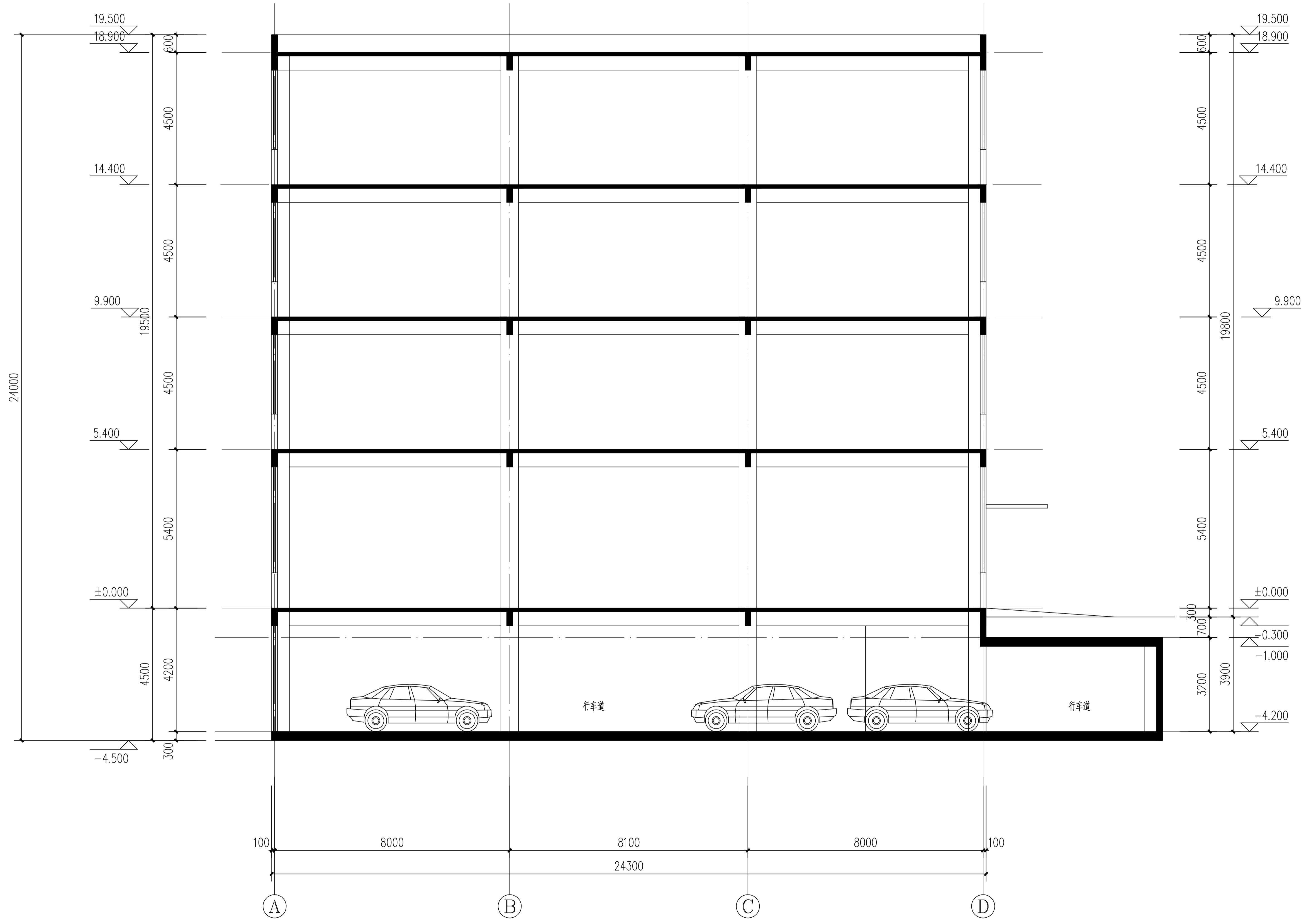
1-1剖面图 1:100
