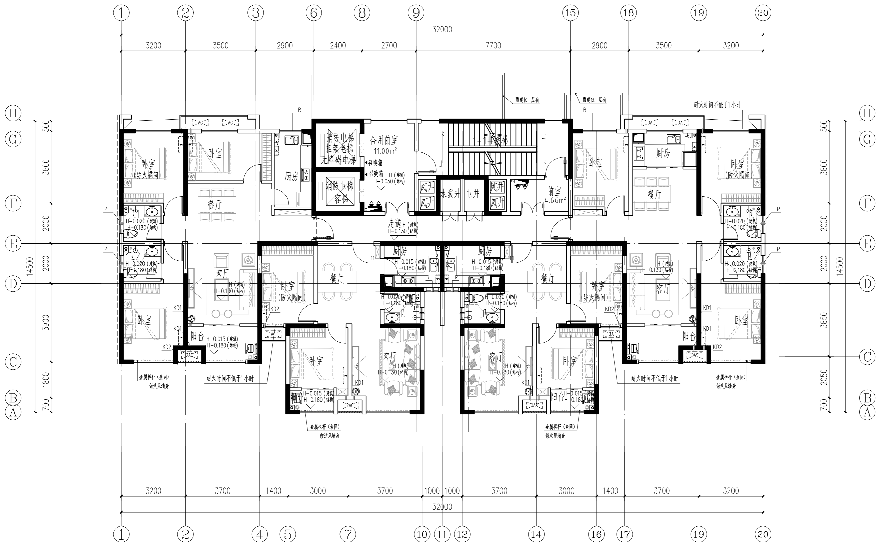
二-二十四层平面图 1:100
