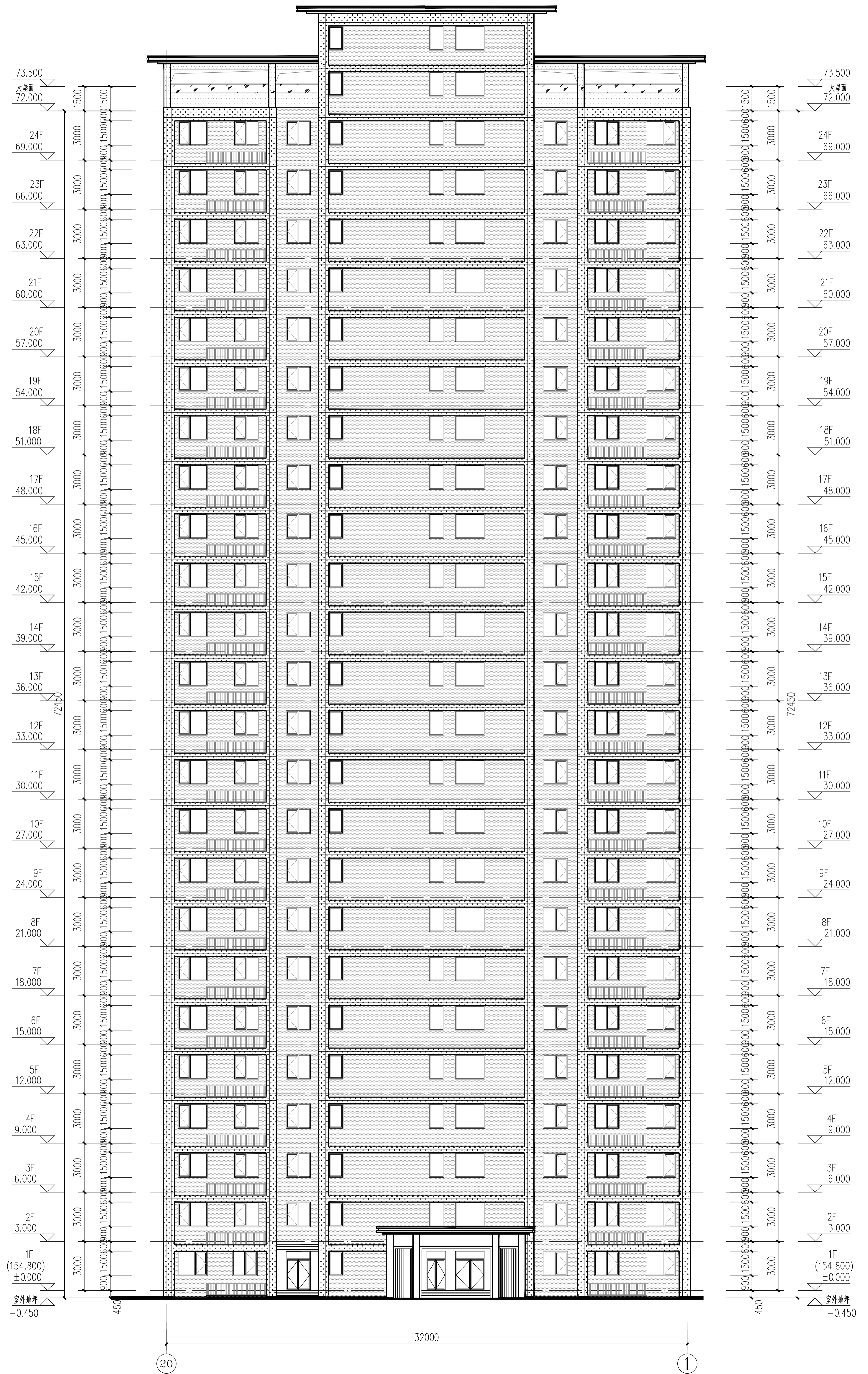
②0-①轴立面图 1:150
