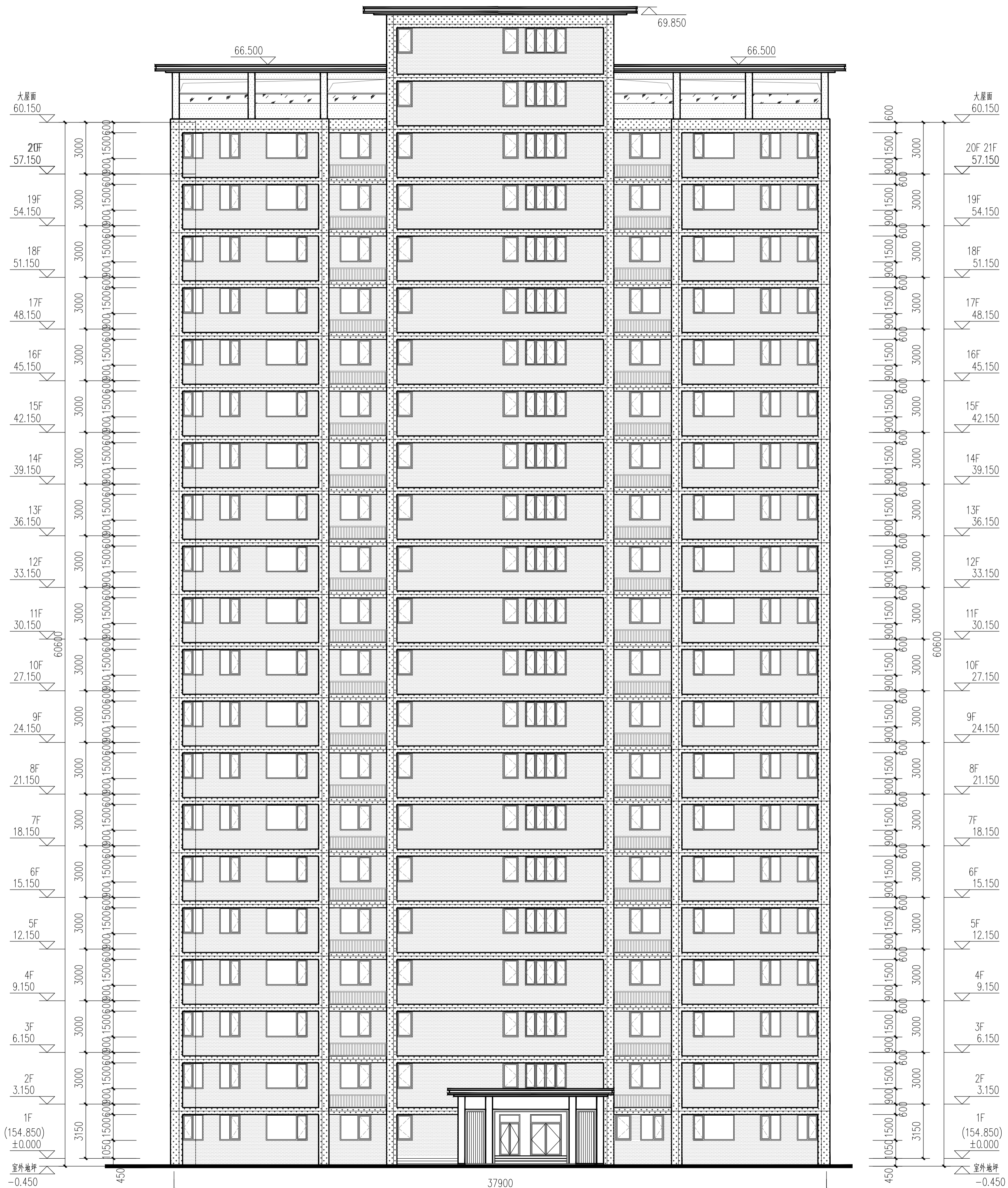
25-①轴立面图 1:150
