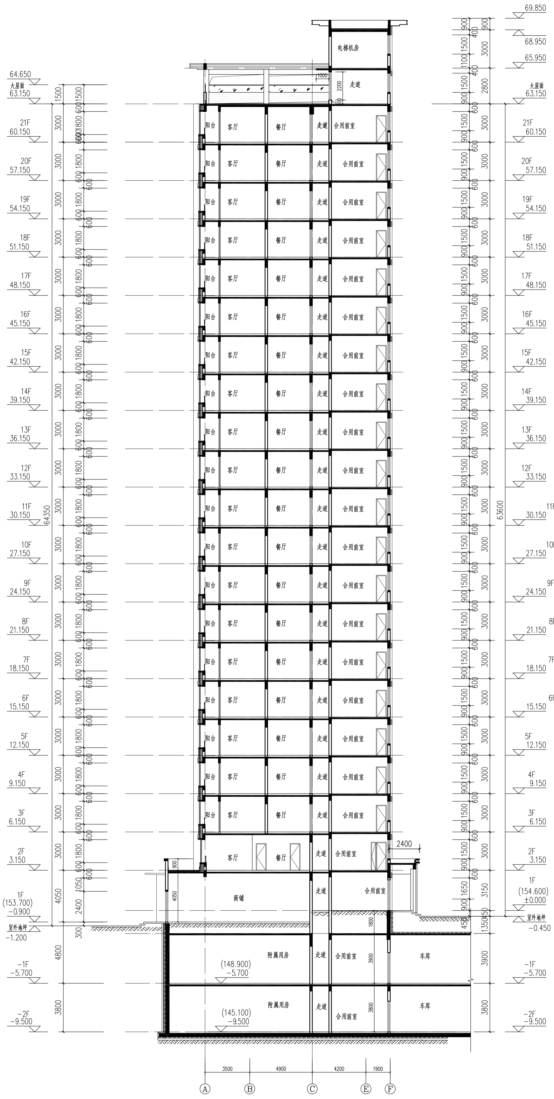
1-1剖面图 1:150
