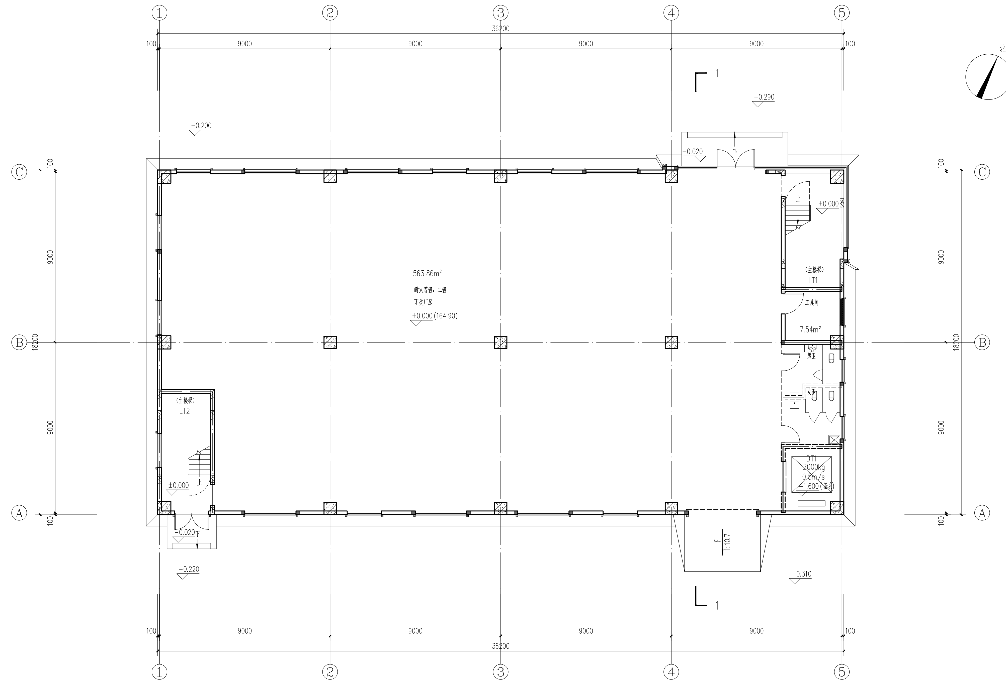
一层平面图 1:100
