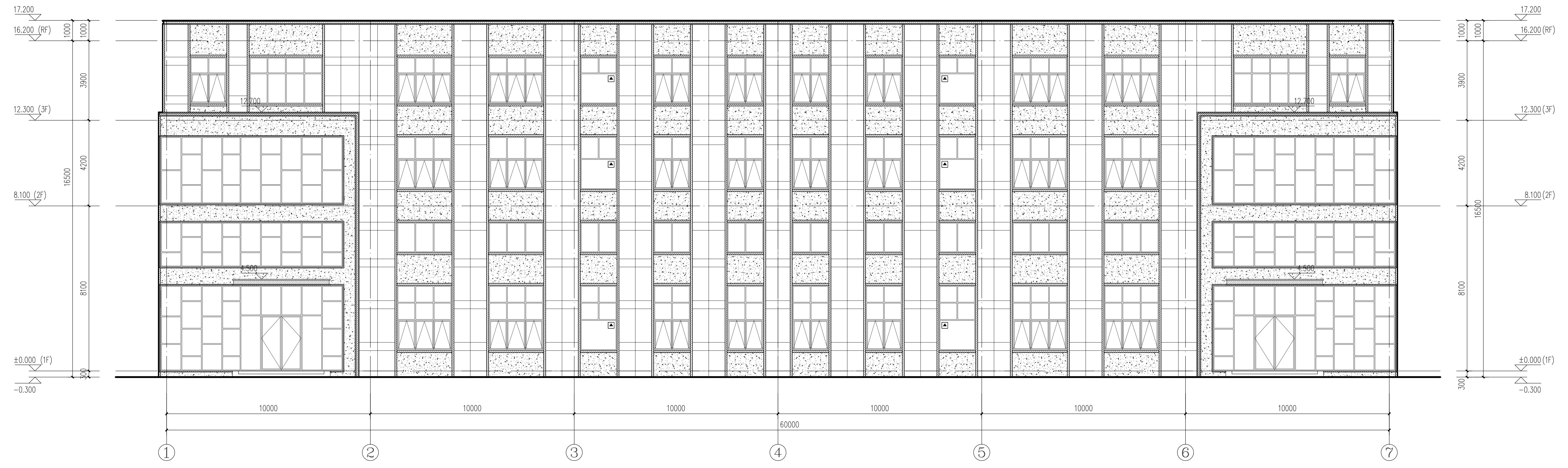
①轴-⑦轴立面图 1:100
