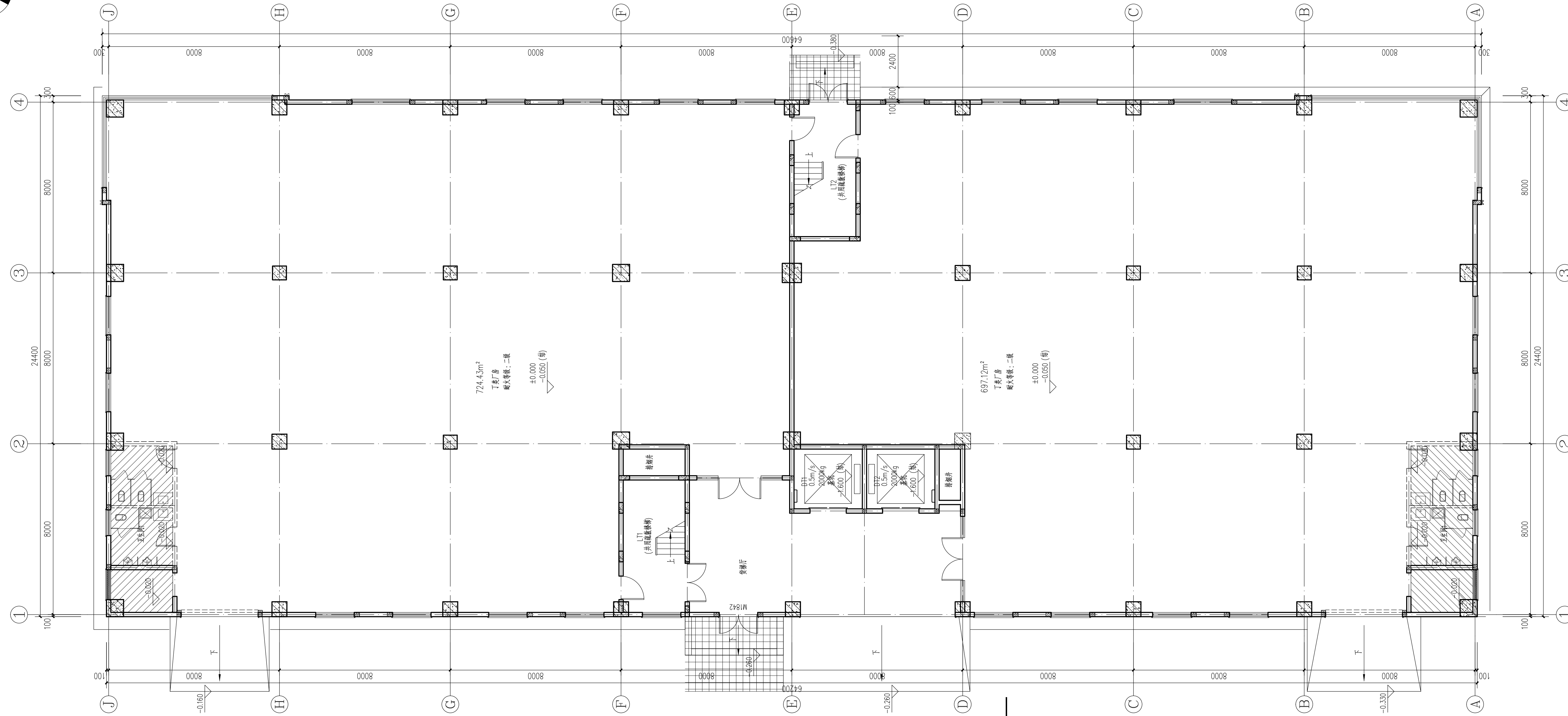
一层平面图 1:100 本层建筑面积: 1562.10m²
