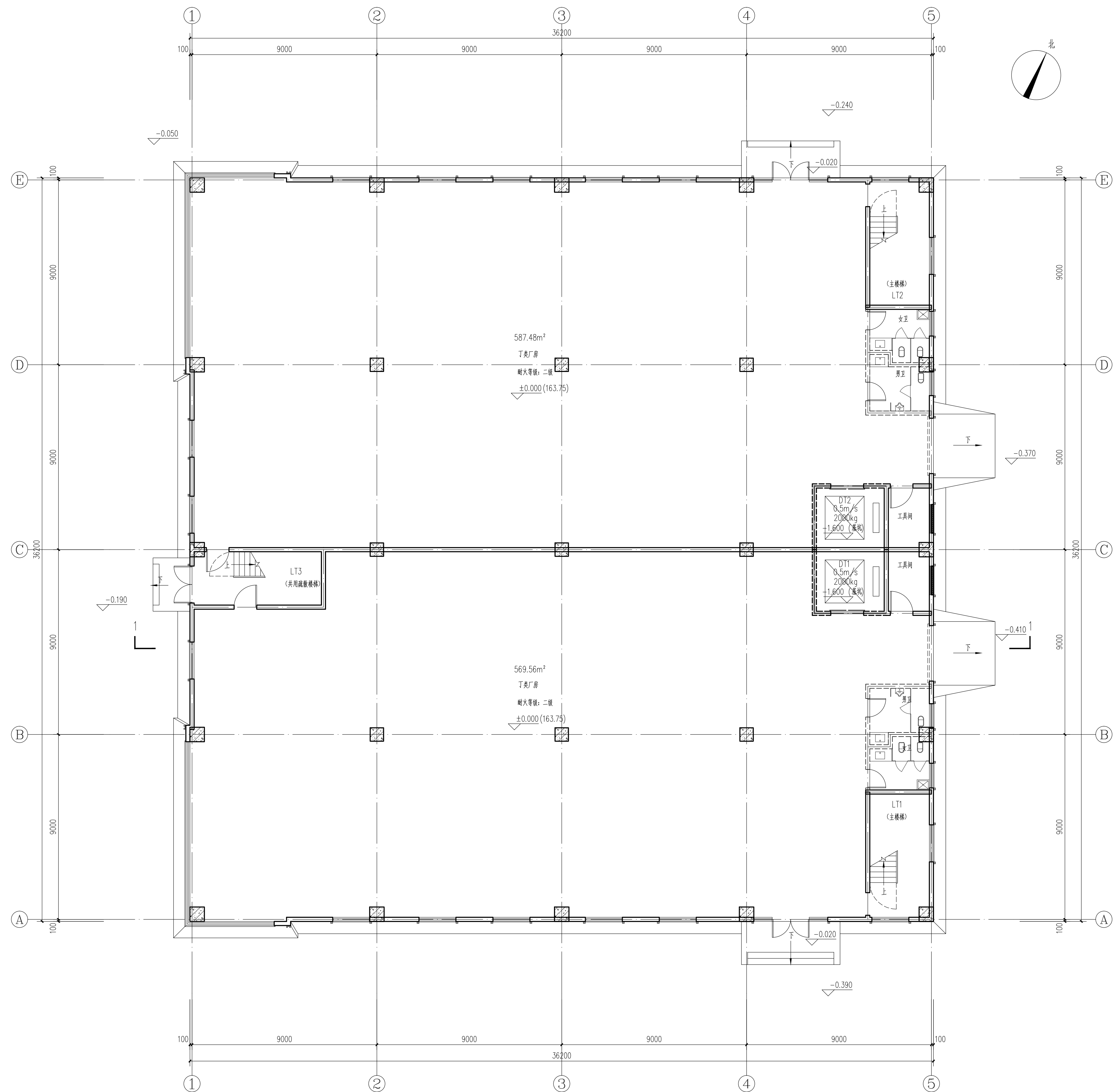
一层平面图 1:100
