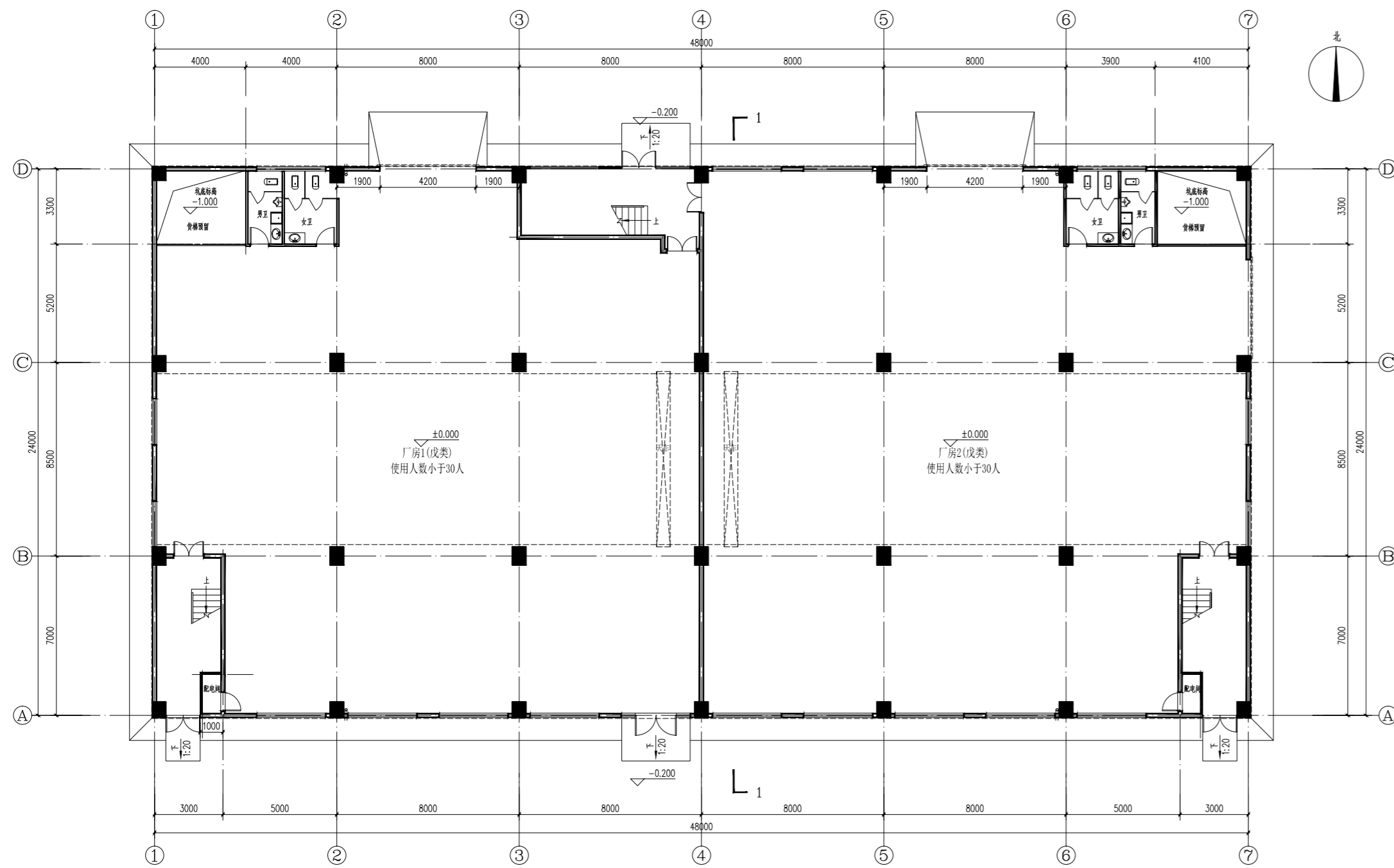
一层平面图 本层建筑面积: 1170.79m 2
