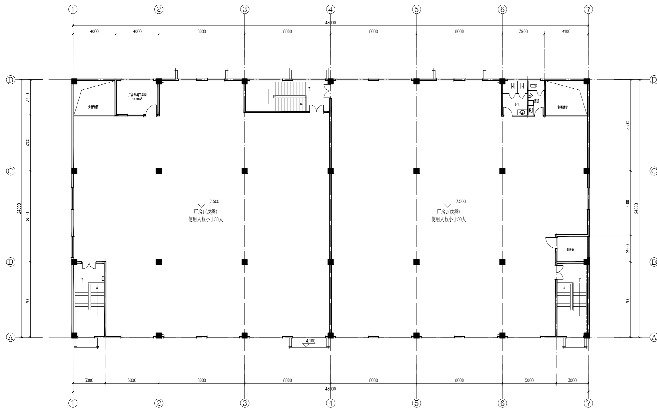
二层平面图 本层建筑面积: 1170.79m 2
