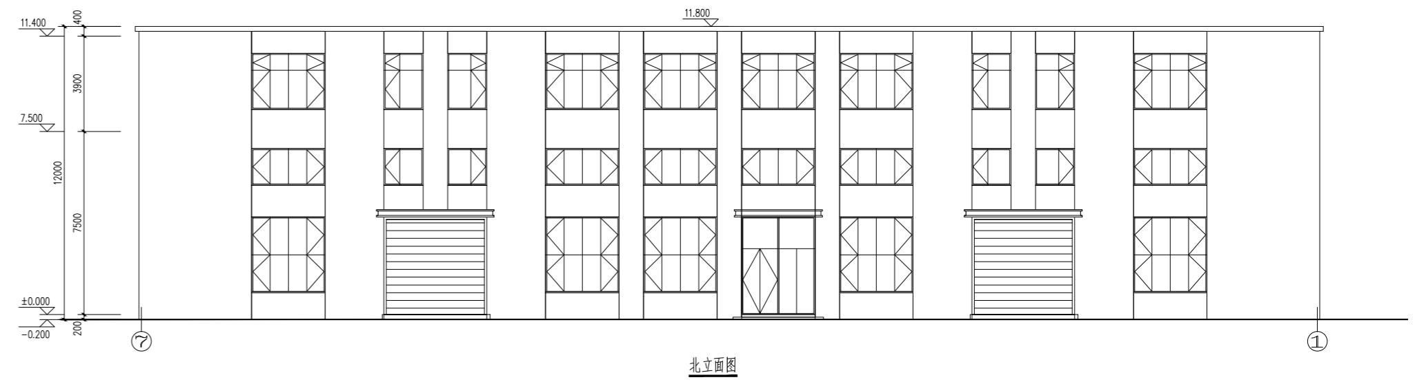
北立面图
