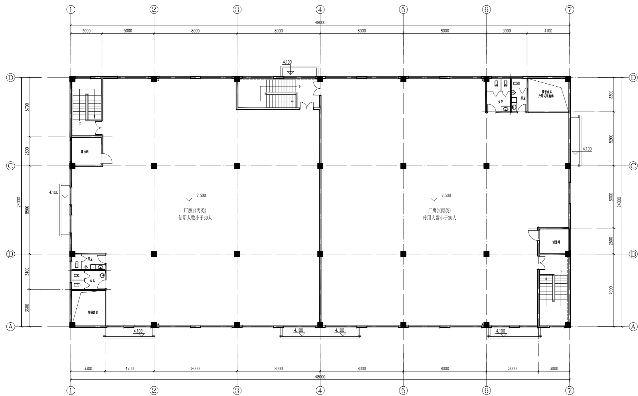
二层平面图
