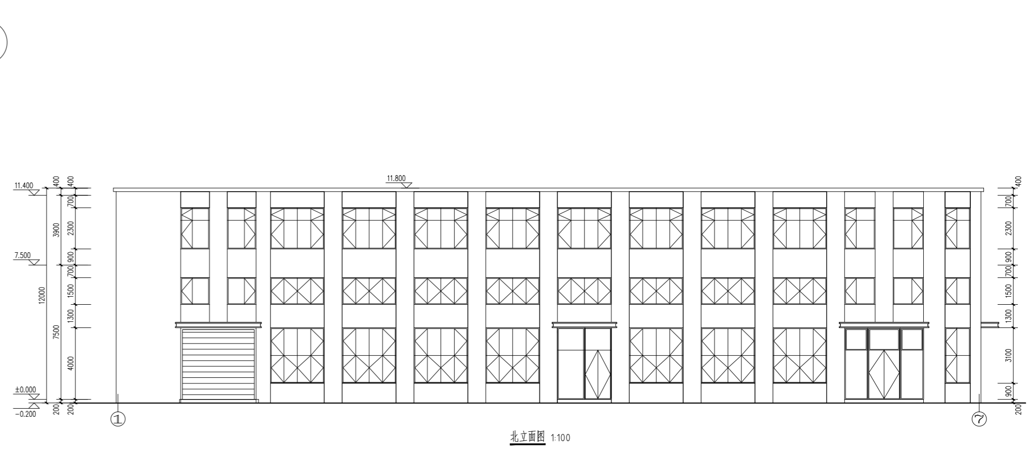
北立面图 1:100
