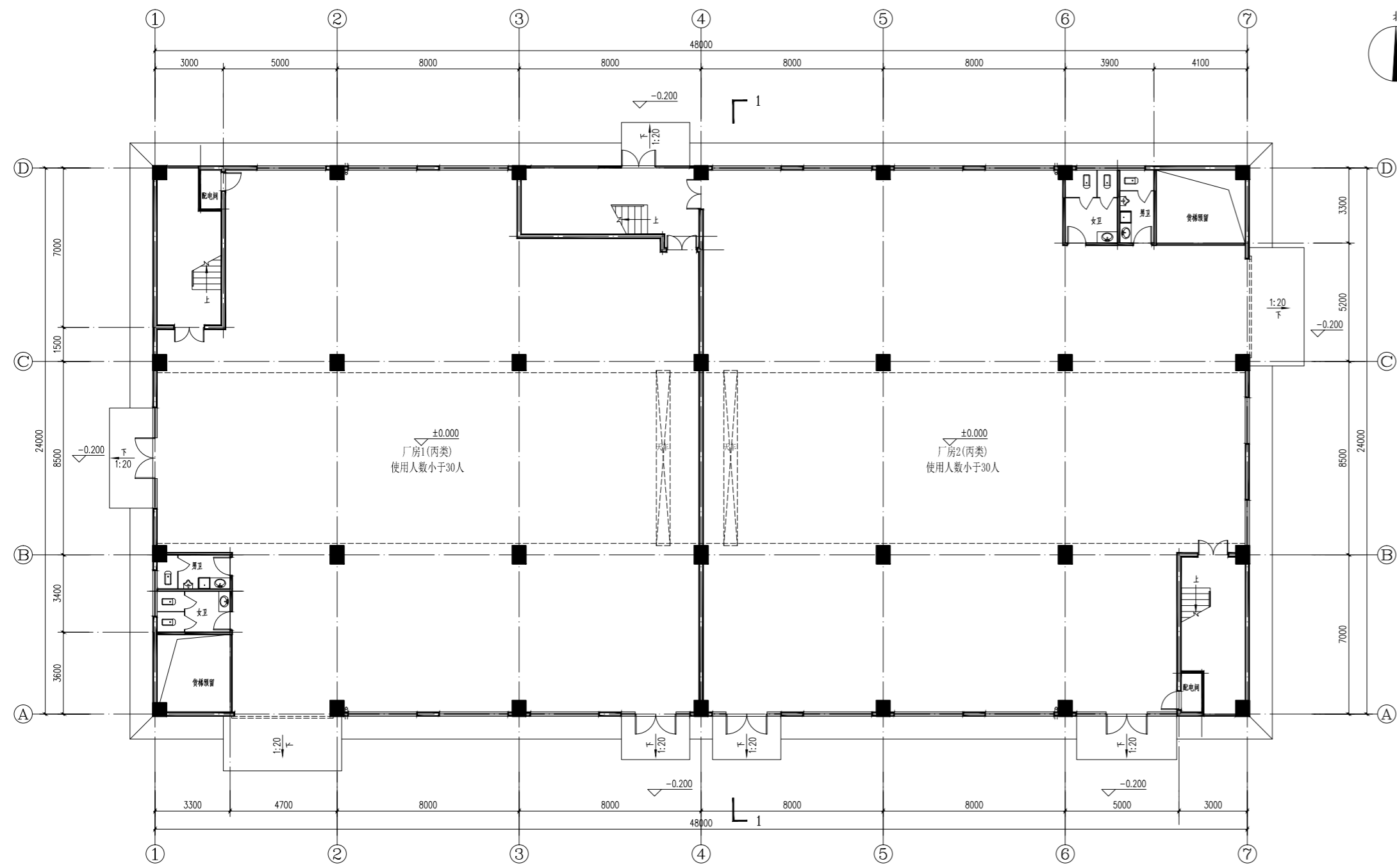
一层平面图
