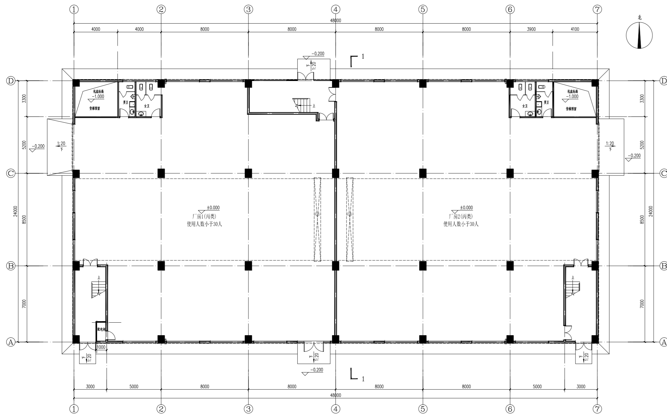
一层平面图
