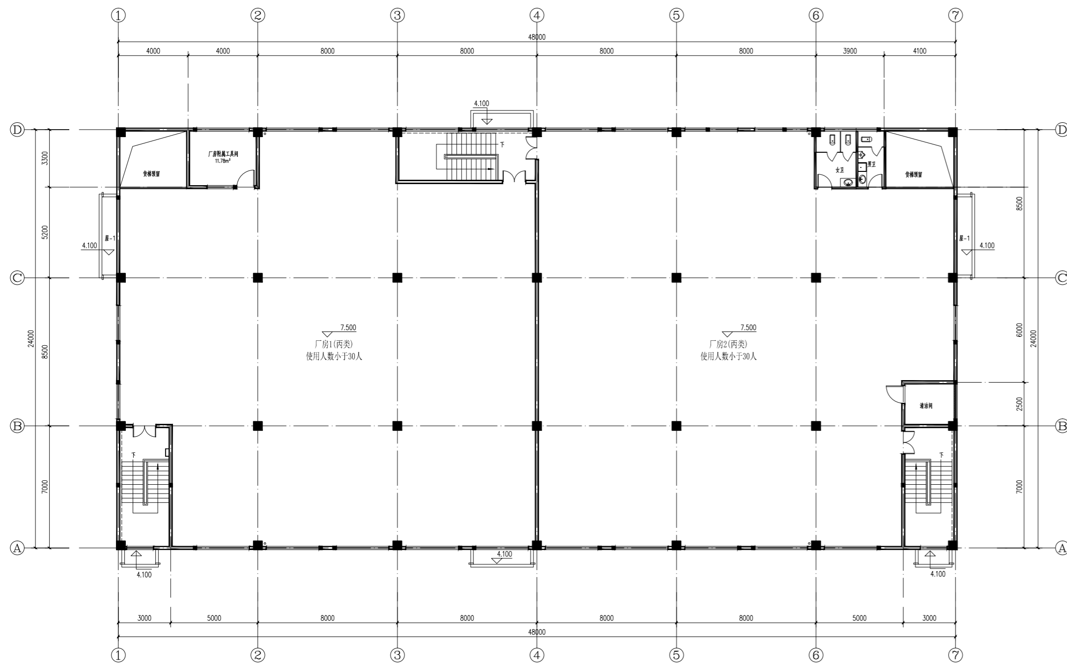
二层平面图
