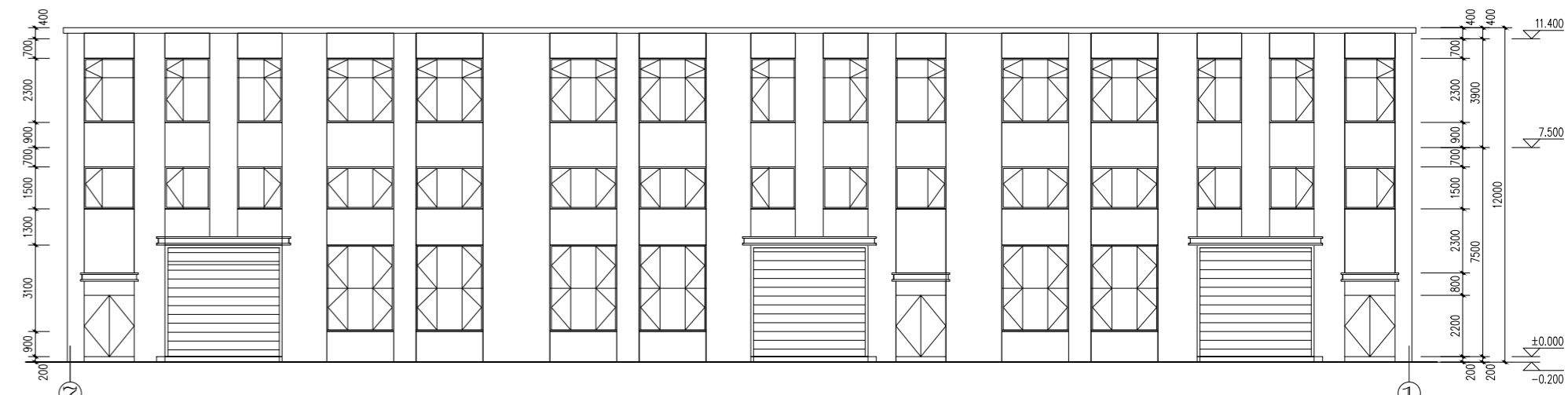
北立面图
