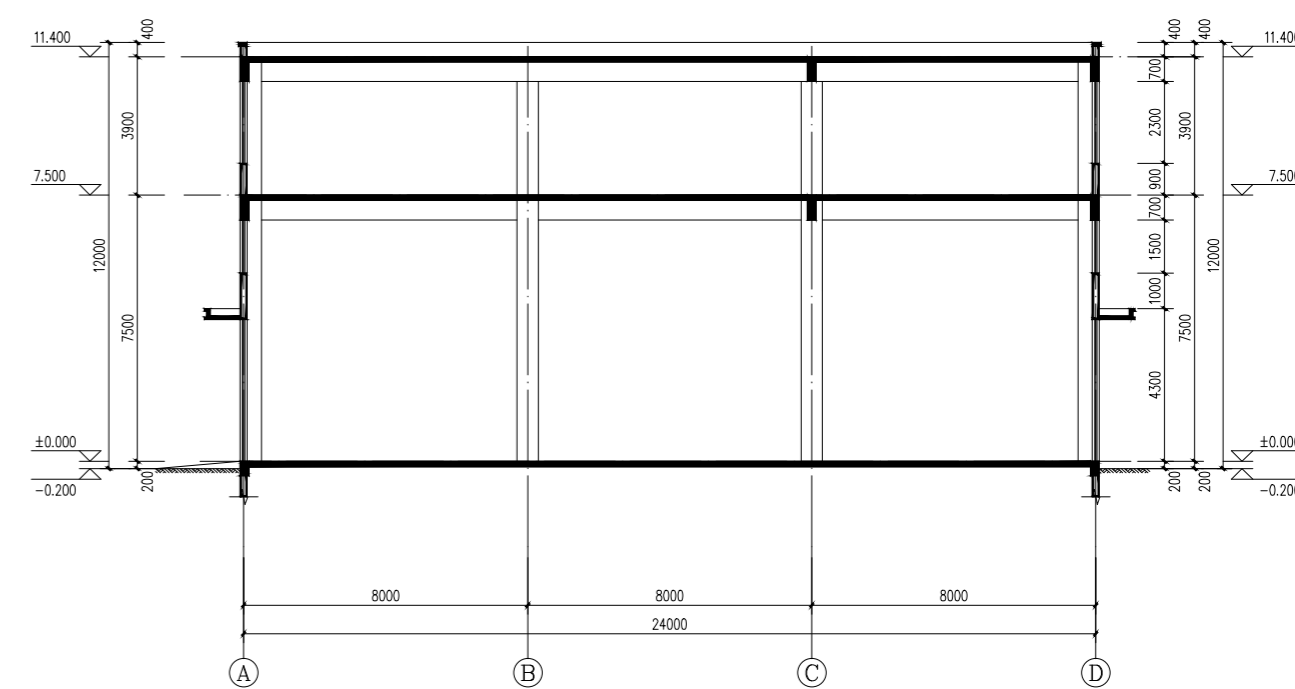
1-1剖面图
