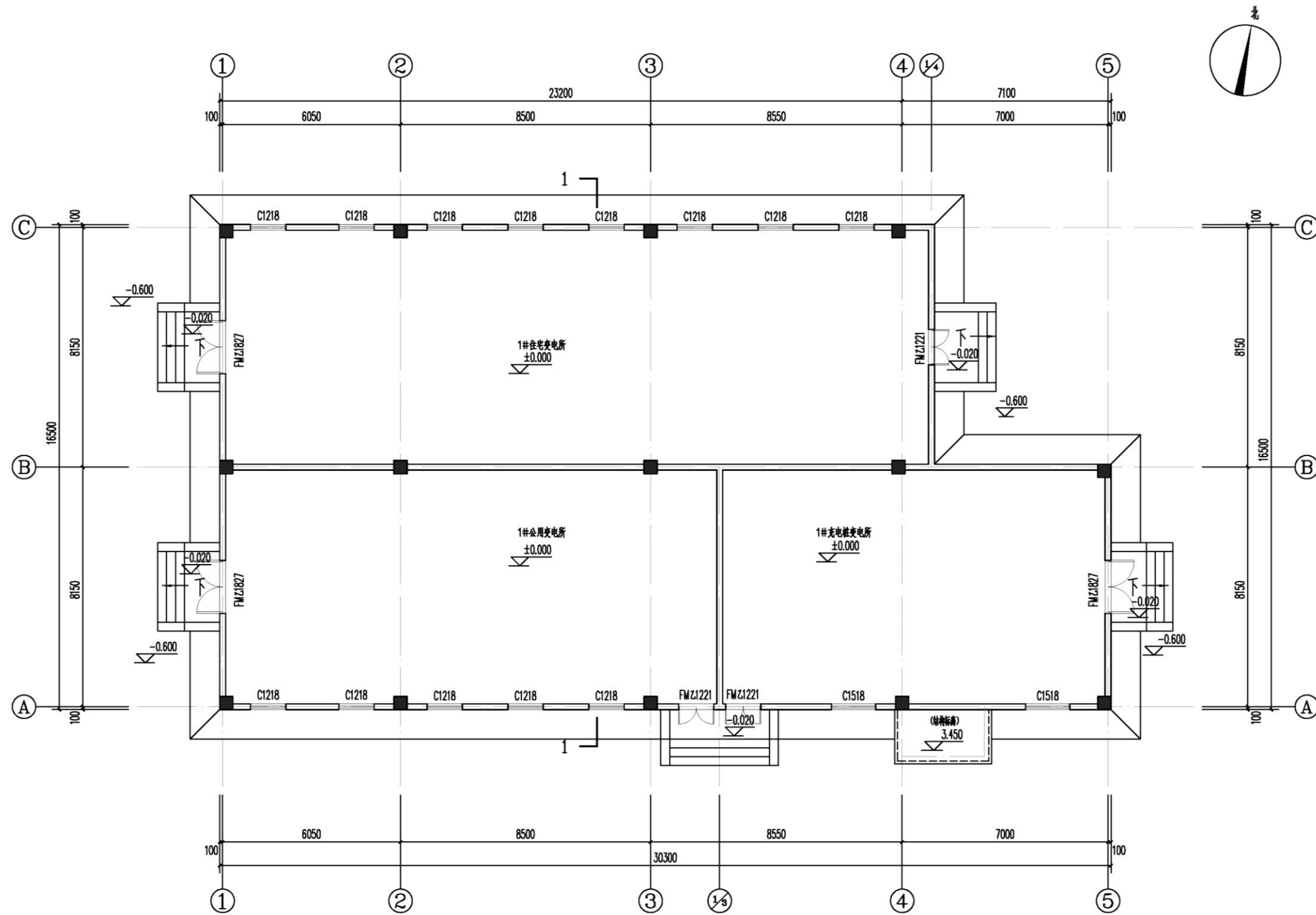
一层平面图 1:100
