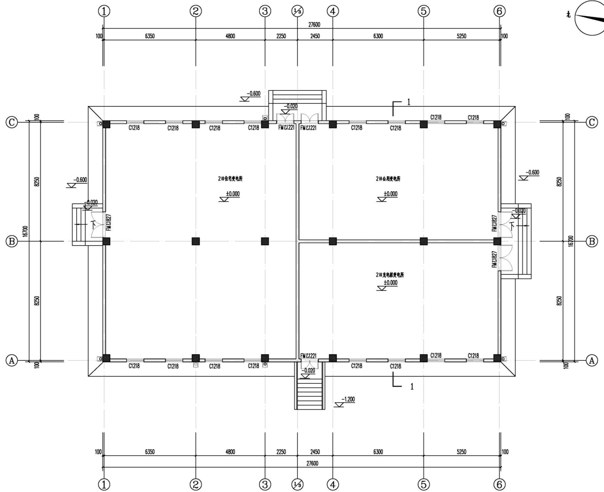
一层平面图 1:100
