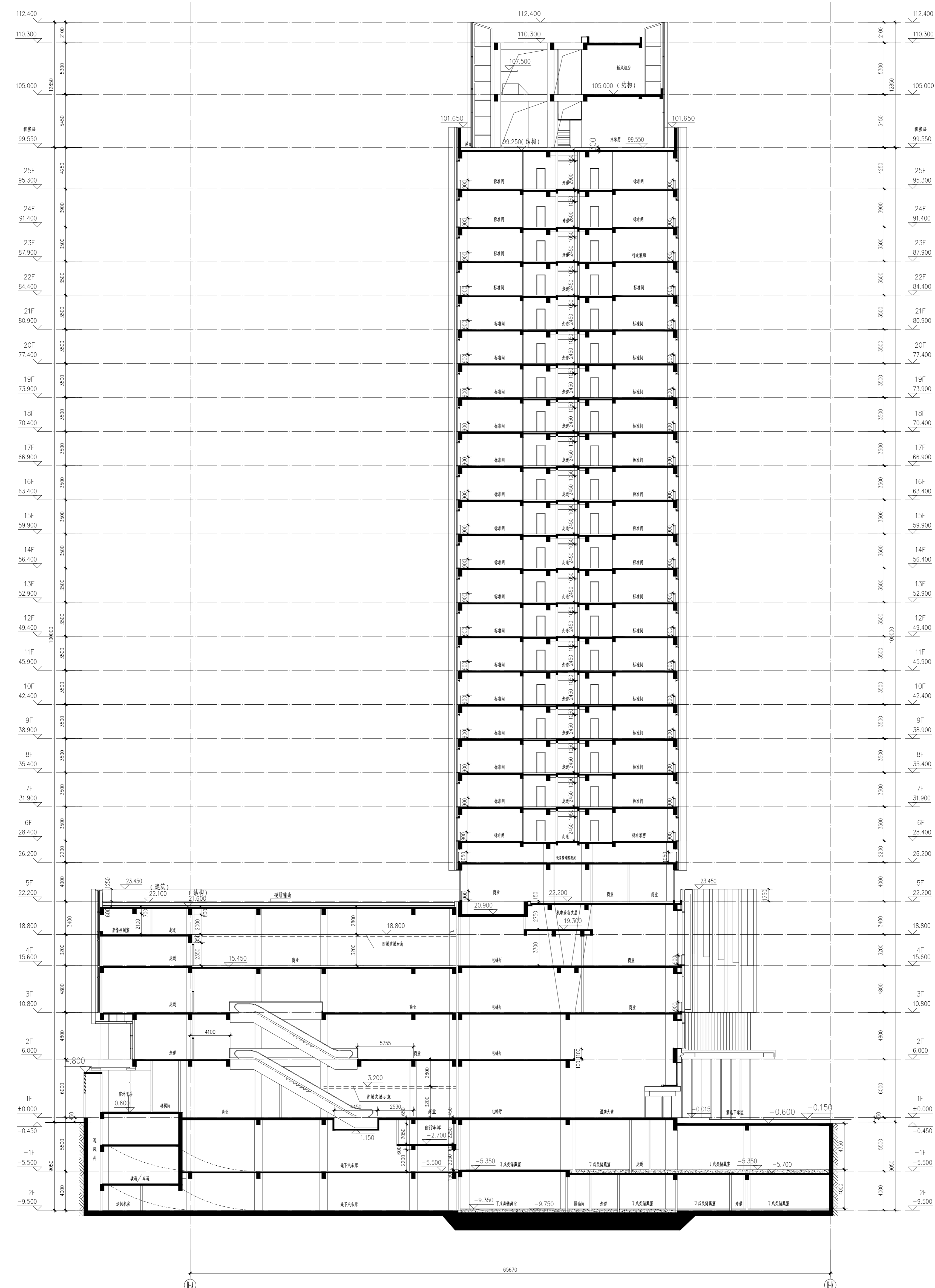
1-1 剖面图
