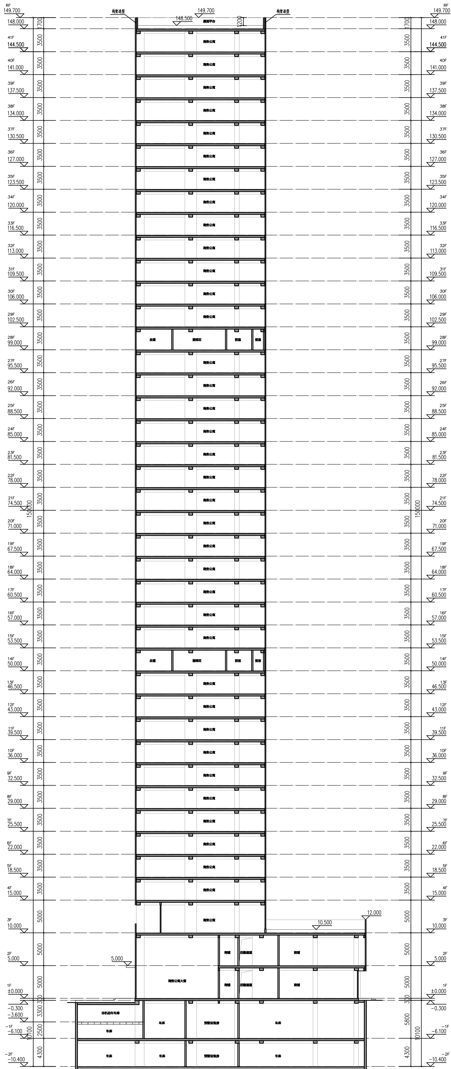
1-1剖面图
